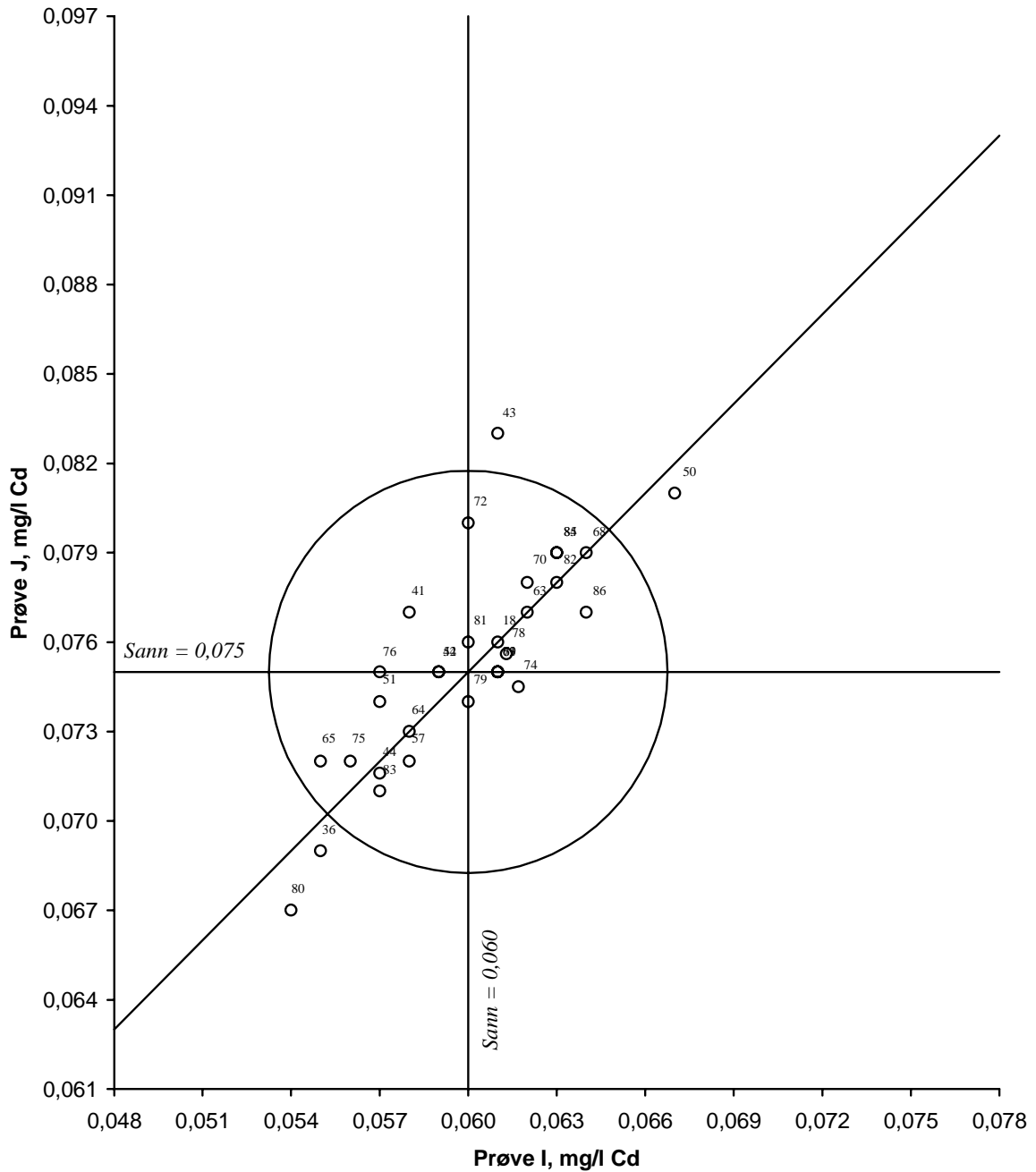
Figur 25. Youdendiagram for kadmium, prøvepar IJ Akseptansgrensen, angitt med en sirkel, er 10 %
