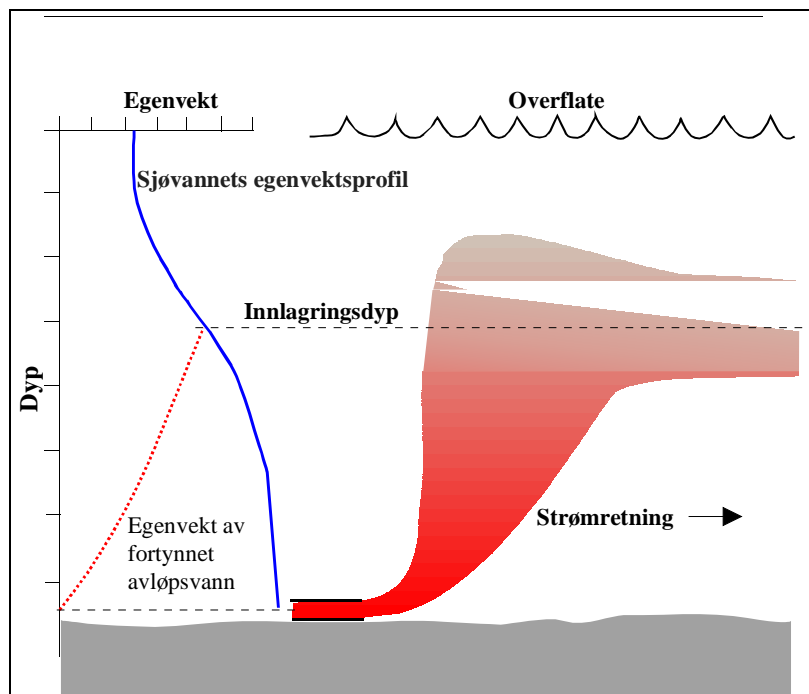
Figur 5. Prinsippskisse av dyputslipp med innlagring av avløpsvann
