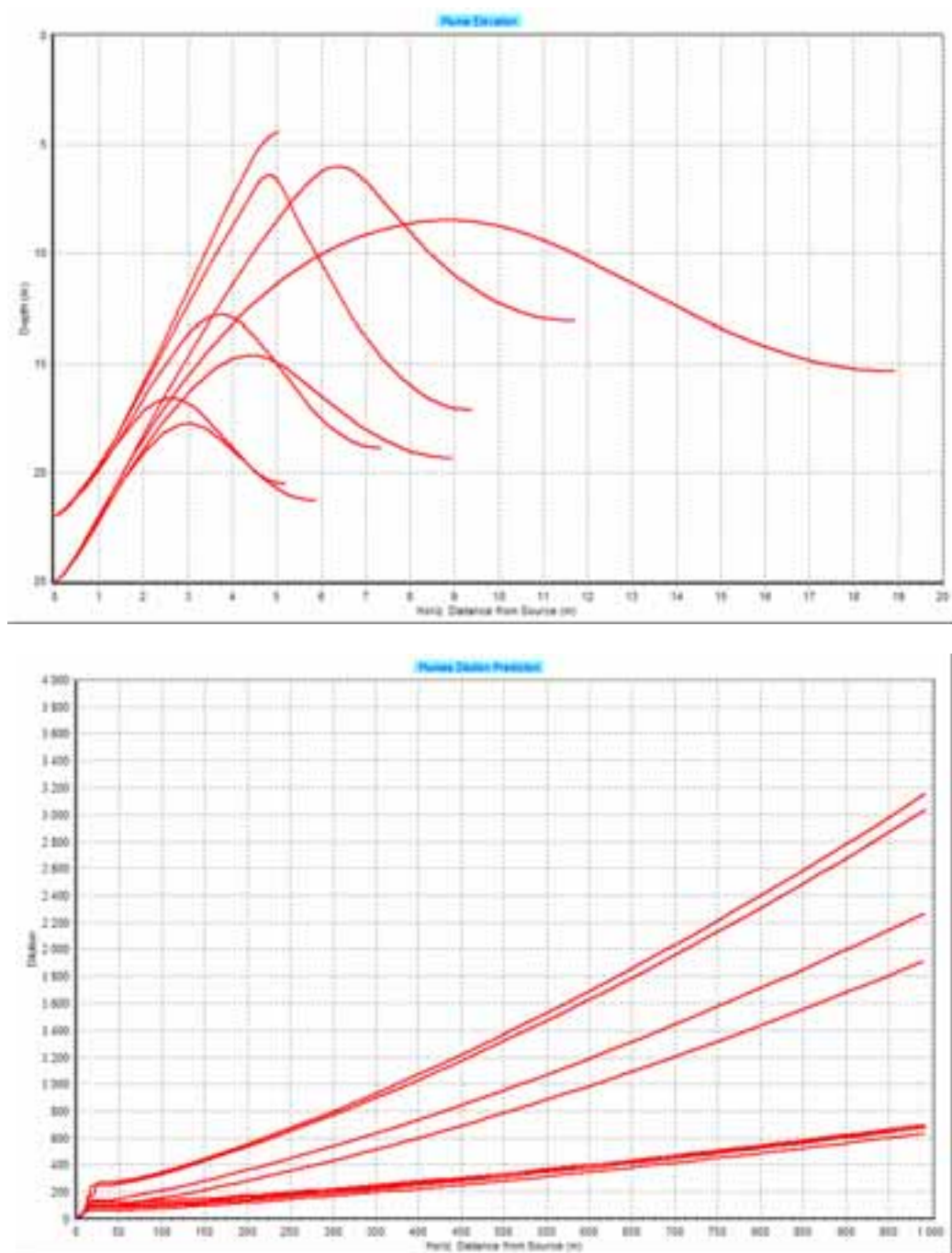
Figur 8. Beregninger for fem utvalgte situasjoner, utslipp i 22 m og 25 m dyp og ved utslipp av 3000 m 3 /s. Strømhastigheten i resipienten er 5 cm/s. Øvre figur viser typisk innlagring for avløpsvannet over diffusoren, med et tilfelle der avløpsvannet innlagres i sprangsjiktet. Nedre figur viser gjennomsnittlig fortynning ved økende avstand fra utslippet.
