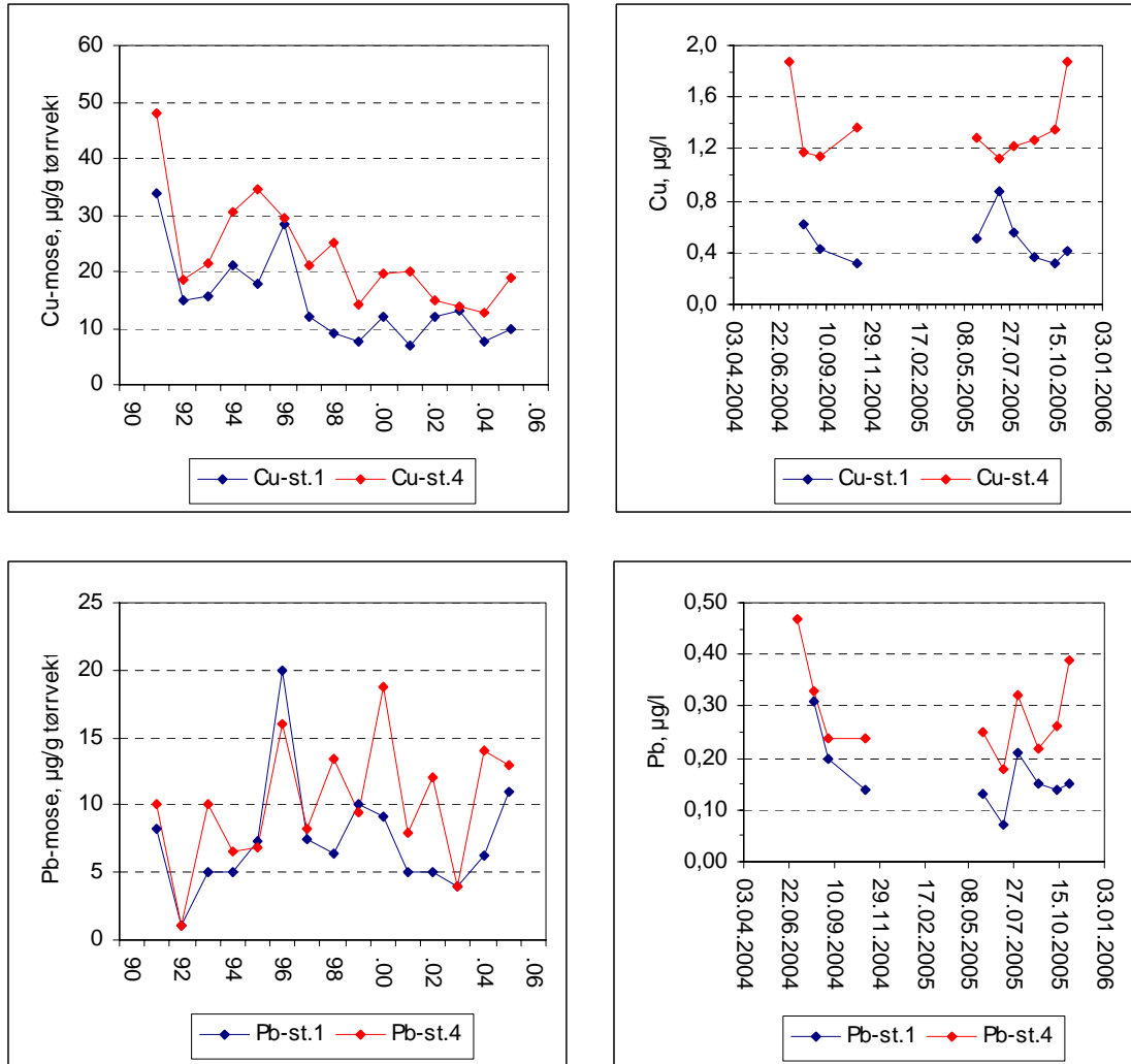
Figur 2. Middeldkonsentrasjonene av kobber (Cu) og bly (Pb) i vannmoser ved stasjon 1 og 4 i Veltmannåa (venstre paneler) og vannkonsentrasjoner av Cu og Pb ved tilsvarende stasjoner i 2004 og 2005 (høyre paneler).
