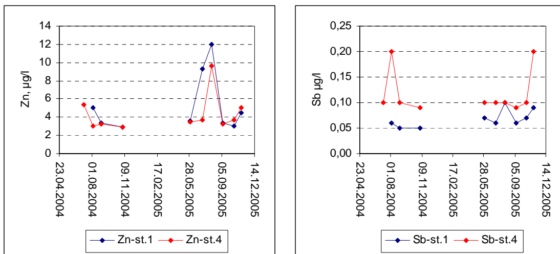
Figur 3. Konsentrasjonene av sink (Zn) og antimon (Sb) i Veltmannåa ved innløp (st.1) og utløp (st.4) av testsenteret.
