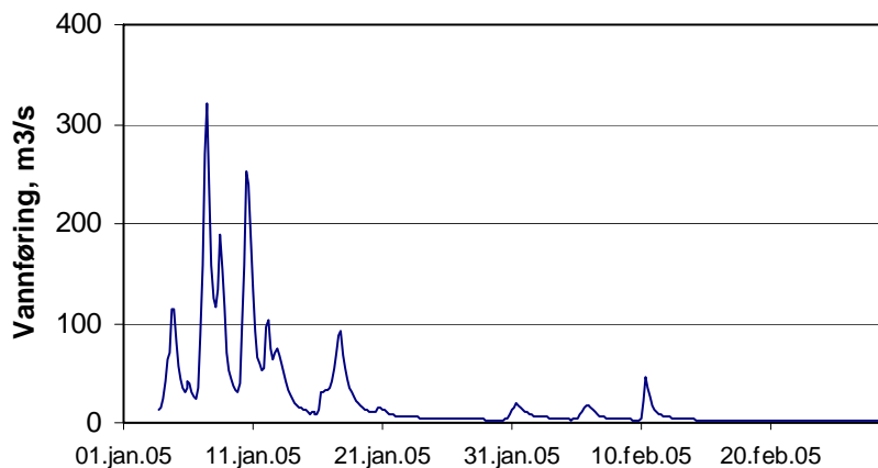
Figur 9. Vannføring (Q) ved Regevik i Sira vinteren 2005. Data fra Sira-Kvina kraftselskap.
