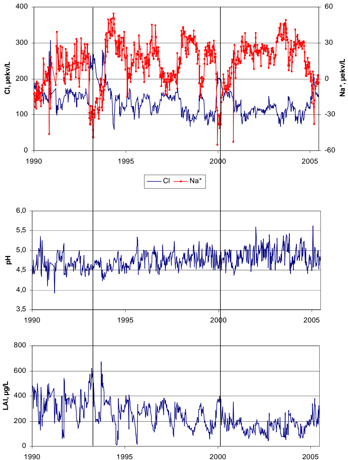
Figur 19. Sjøsaltepisoder i Birkenes i perioden 1990 - juli 2005. Episodeindikatorerne Cl og ikke-marin Na (Na*) er vist øverst, mens effektene på pH og labilt Al er vist under. Vertikale hjelpelinjer markerer episodene vintrene i 1993 og 2000, se også Tabell 2 .
