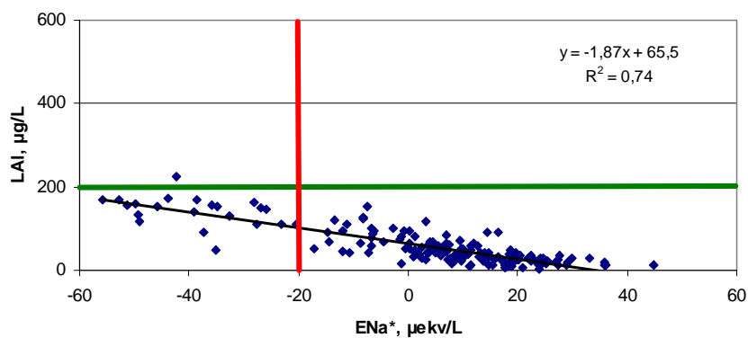
Figur 21. Forholdet mellom sjøsaltindikatoren ikke-marin Na ( Na^* ) og LAI i Birkenesfeltet (de to øverste figurene) og Øygardsbekken (to nederste). Alle data i perioden januar 1990-mai 1995 er sammenliknet med data for perioden november 1999-juni 2005 i Birkenes, mens data for mai 1992 - mai 1998 er sammenliknet med data fra mai 1998-juni 2005 i Øygardsbekken. Vertikal hjelpelinje markerer Na^* = -20 µekv/L, mens horisontal hjelpelinje er ved hhv. 400 og 200 µg LAI/L.
