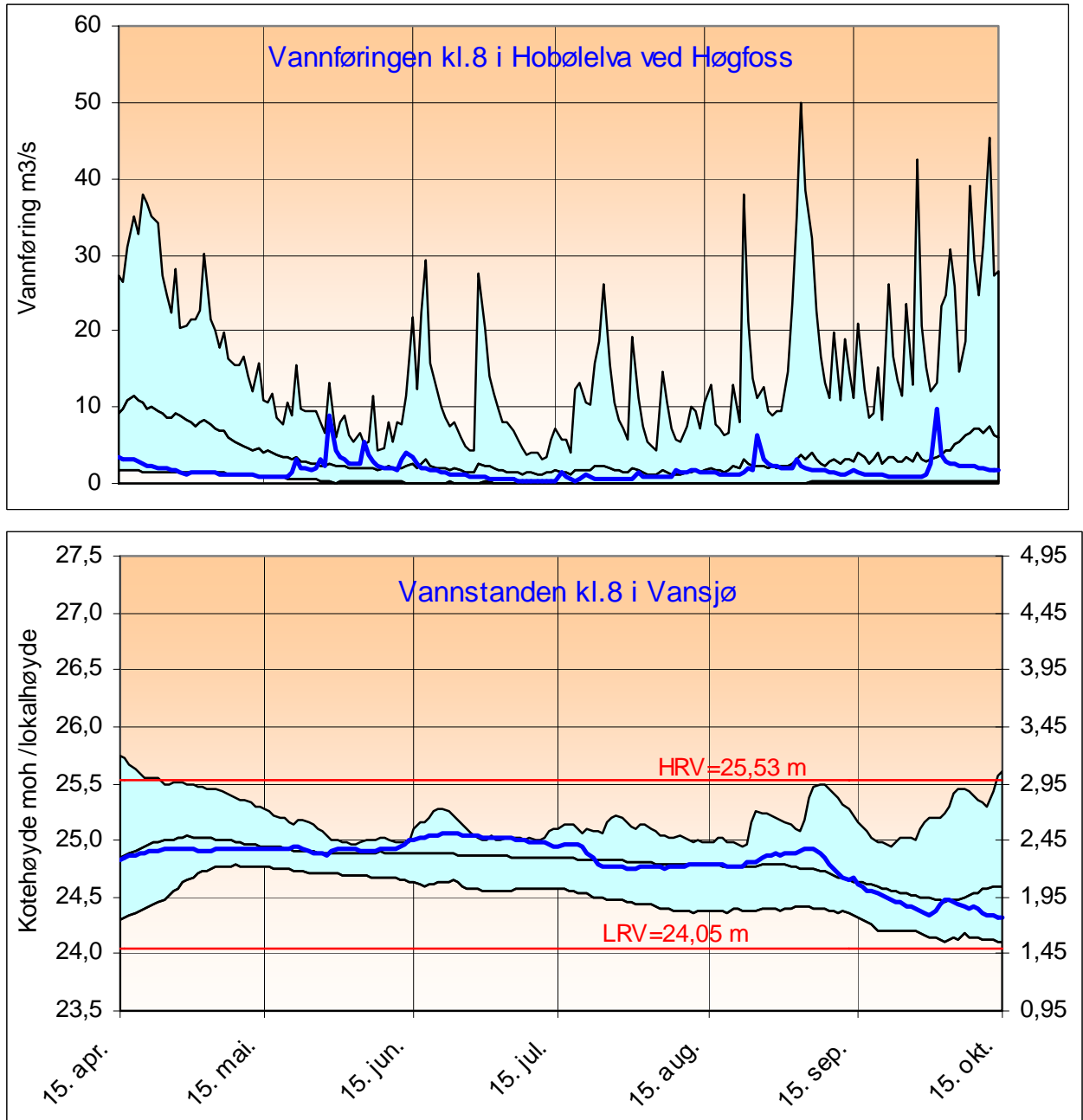
Figur 6. Vannføring i Høbølelva v/Høgfoss og vannstand i Vansjø v/ Vanemfjorden nord. Blå kurve viser årets data. "Bakgrunnsteppet" er maksimum, middel og minimum for årrekken 1983-2004 (Kilde: Glommen og Laagens Brukseierforening, http://www.glb.no , se forøvrig http://82.147.36.230/default/Public/MB/Mossevassdraget.htm der oppdatert informasjon foreligger)
