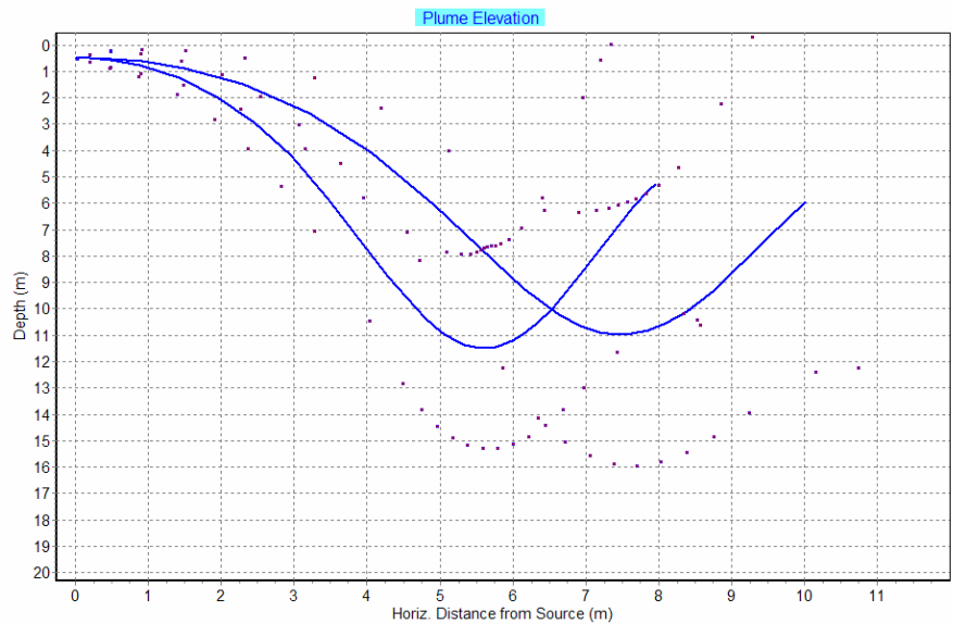
Figur 4. Simulering av utslipp ved strømhastighet 2 cm/s. Den øvre figuren viser innlgringsdyp ved vannmengden 3 m 3 /s og 4,5 m 3 /s. For begge vannmengder sank først kjølevannet ned til 10-12 m dyp, men innlagret seg deretter i ca. 4-8 m dyp.
