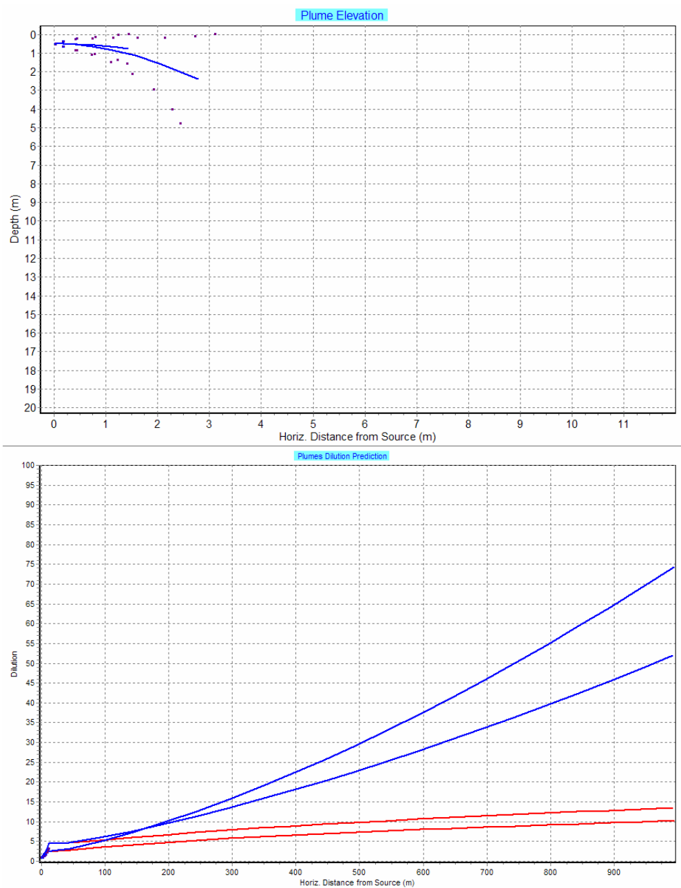
Figur 6. Simulering av utslipp ved strømhastighet 10 cm/s. Innlagringsdyp (øverst) og fortynning (nederst) ved vannmengder 3 \text{ m}^3/\text{s} og 4,5 \text{ m}^3/\text{s} . Kjølevannet synker ikke så langt som i tilfellet er ved svak strøm, men innlagres sannsynligvis i 5-6 m dyp (øvre del av sprangsjiktet, jfr. Figur 3 ). Beregningene av fortynning er utført med konstant turbulent blandingskoeffisient (to røde kurver i nedre figur) og koeffisient som øker med avstanden (blå kurver i nedre figur).
