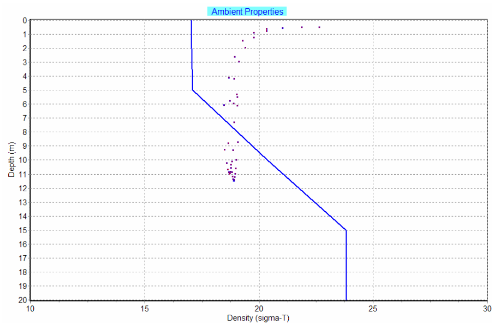
Figur 3. Simulering av utslipp ved strømhastighet 2 cm/s. Heltrukken linje viser den vertikale sjiktningen (vannets egenvekt gitt ved størrelsen sigma-t) den 6.11.2005, og den stiplede kurven viser hvordan kjølevannets egenvekt avtok fra det ble sluppet ut i overflatelaget og mens den sank nedover og blandet seg med sjøvannet. Likevekt ble oppnådd omkring 8 m dyp. Figuren bør sees i sammenheng med Figur 2 og Figur 4 .
