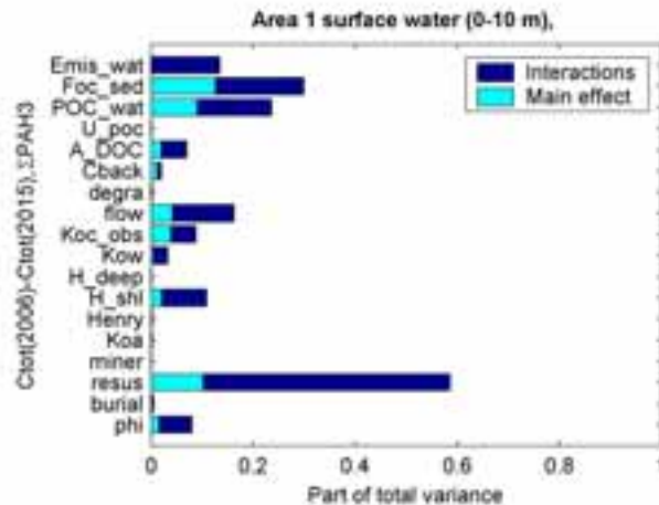
Figur 8. Følsomhetsanalyse av modellresultater i Ranfjorden. “Main effect” viser parameterens egen effekt og “Interactions” effekten med andre parametre. Det analyserte modellresultatet er her reduksjonen i total vannkonsentrasjon av PAH i Area 1 (0-10 m) fra 2006 til 2015, antatt en 50 % reduksjon i landbaserte emisjoner i 2007. Parameterforkortelser og verdi-intervaller er forklart i Tabell 1, bortsett fra for “Emis_wat” (landbaserte emisjoner til vann) som har en verdi-intervall på 100-1000 kg/år.
