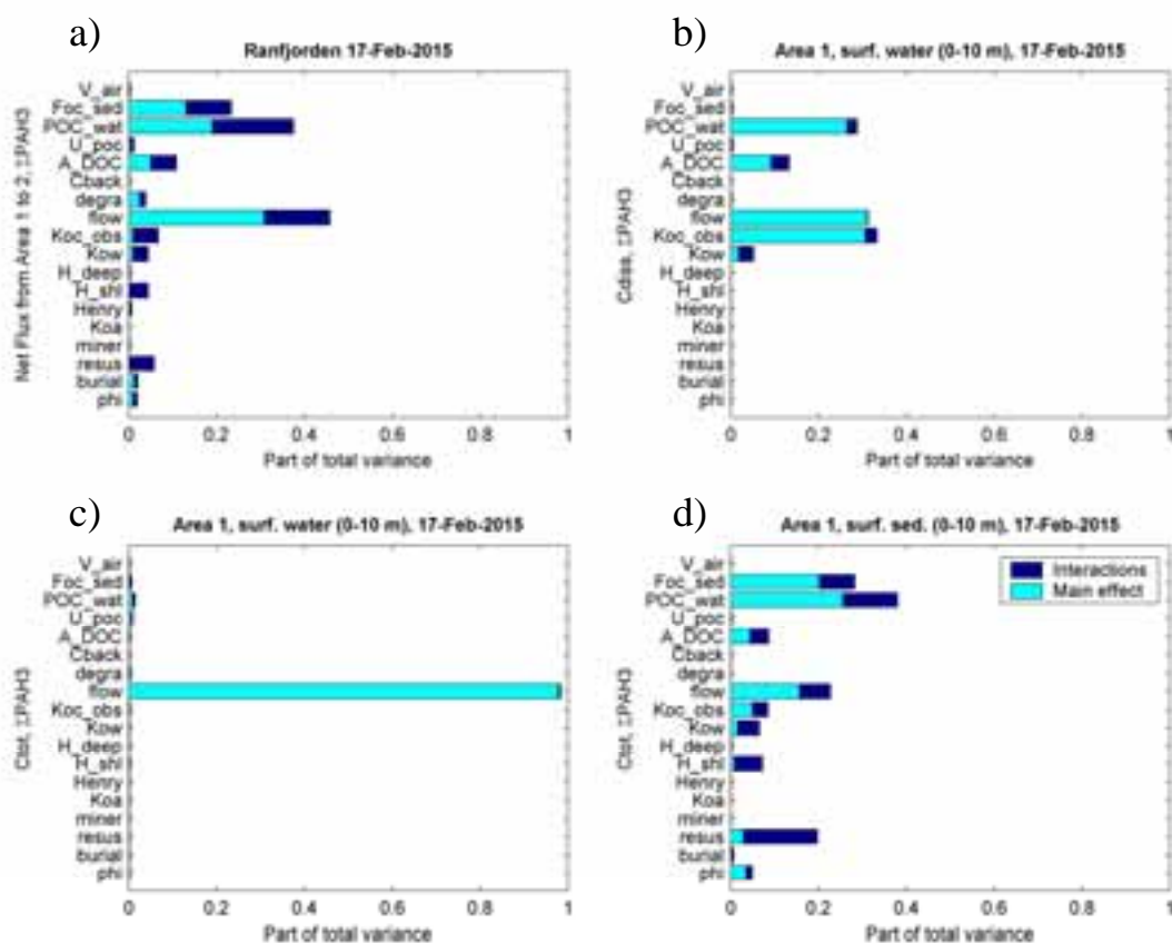
Figur 4. Følsomhetsanalyse av modellresultater i Ranfjorden. “Main effect” viser parameterens egen effekt og “Interactions” effekten med andre parametere. De studerte modellresultater er (a) PAH-fluksen fra Area 1 til 2, (b) løst og (c) total PAH-konsentrasjon i 0-10 m vannkolonne i Area 1, og (d) total PAH-konsentrasjon i 0-10 m sedimentområde i Area 1 i år 2006 (figuren på forrige side) og 2015 (figuren på denne siden). Parameterforkortelser er forklart i Tabell 1.
