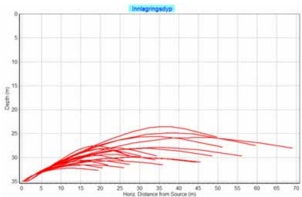
Figur 10. Innlagringsdyp ved utslipp i 35 m dyp når vannmengden er 10, 20 og 40 l/s og strømhastigheten 10 cm/s. Innlagringsdypet er ca. 25-32 m.
