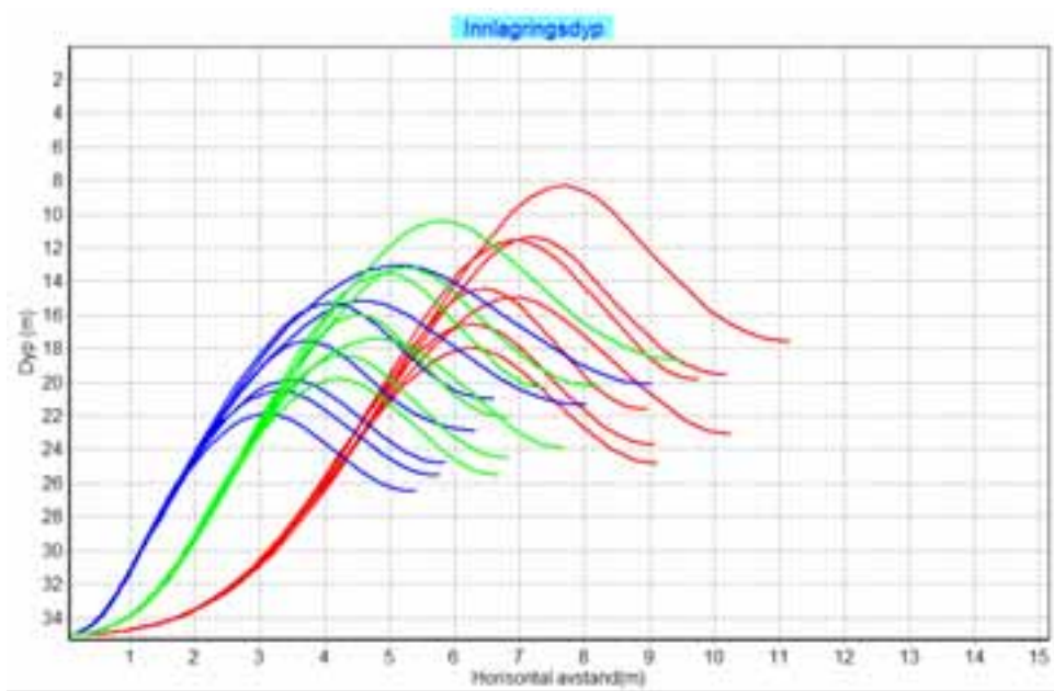
Figur 12. Innlagringsdyp ved utlipp i 35 m dyp når vannmengden er 10 l/s (blå linjer), 20 l/s (grønne linjer) og 40 l/s (røde linjer) og strømhastigheten 2 cm/s. Figuren viser "strålebanene" for de 9 vertikallprofilene. Innlagringsdypet varierer mellom ca. 16-26 m.
