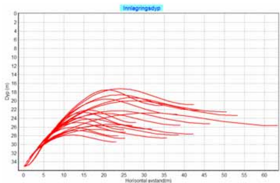
Figur 13. Innlagringsdyp ved utlipp i 35 m dyp når vannmengden er 10, 20 og 40 l/s og strømhastigheten 10 cm/s. Innlagringsdypet er ca. 20-30 m.
