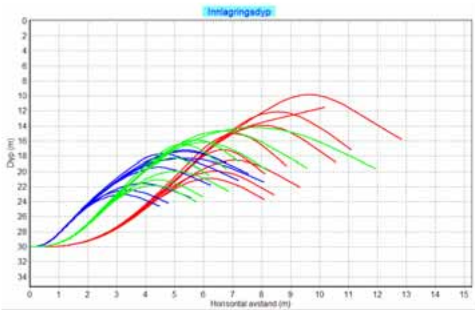
Figur 11. Innlagringsdyp ved utslipp i 30 m dyp gjennom en diffusor med 7 hull med diameter 7 cm og innbyrdes avstand 2,5 m. Vannmengden er 10 l/s (blå linjer), 20 l/s (grønne linjer) og 40 l/s (røde linjer) og strømhastigheten 2 cm/s. Innlagringsdypet er ca. 15-25 m.
