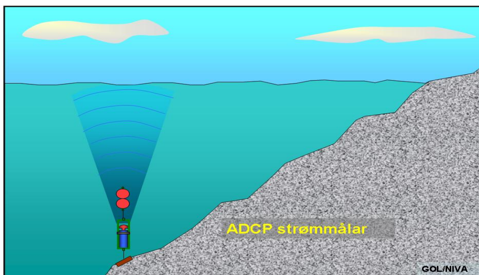
Figur 21. Skisse av strømmålar i posisjon (Kvernevik/Flesland). Ankeret var på 40 m djup, målareren stod eit par meter over dette. Akustiske signal dekkja sjikt frå nær målareren til opp mot overflata, med data frå 10 nivå (djupneceller).
