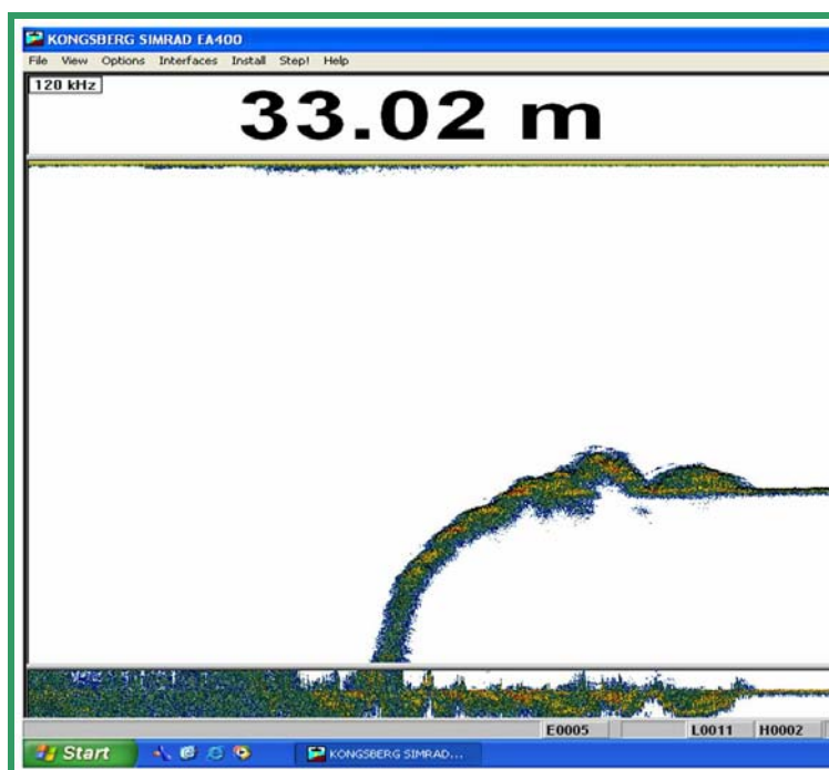
Figur 37. Ekkolodd-snitt frå Kverneviken, frå kanten vestafor diffusoren og over ”knekken” inn på plataet (33 m djup) t.h. i biletet.
