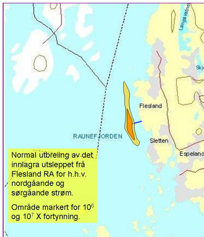
Figur 62. Horisontalfordeling av normal utbreiing av det fortynna og innlagra utsleppsvatnet frå Flesland RA, for nordgåande og sørgåande strøm. Blå strek indikerer avlaupsrøyret. Skya vil typisk representere vatn frå 10 til 17-18 m djup.
