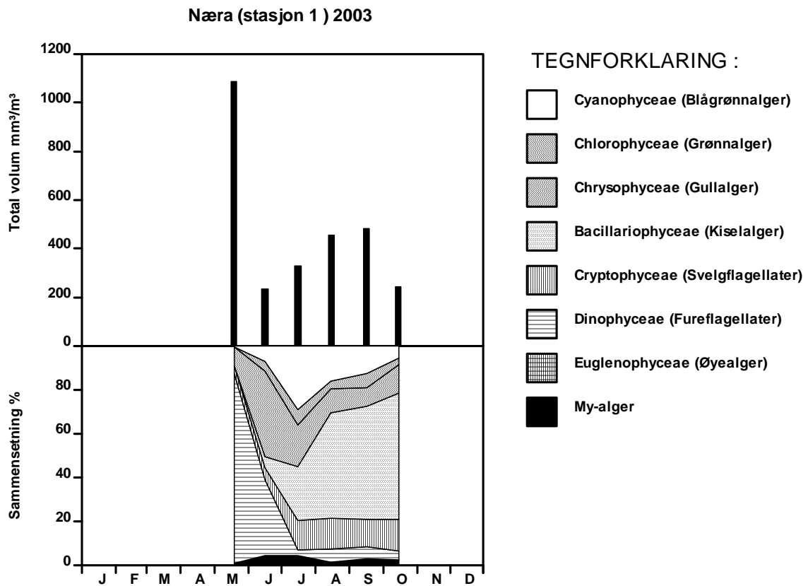
Figur 5. Variasjon i totalvolum, biomasse og sammensetning av planteplankton i Næra i vekstperioden 2003. Totalvolum gitt i mm 3 /m 3 = mg våtvekt/ m 3 .
