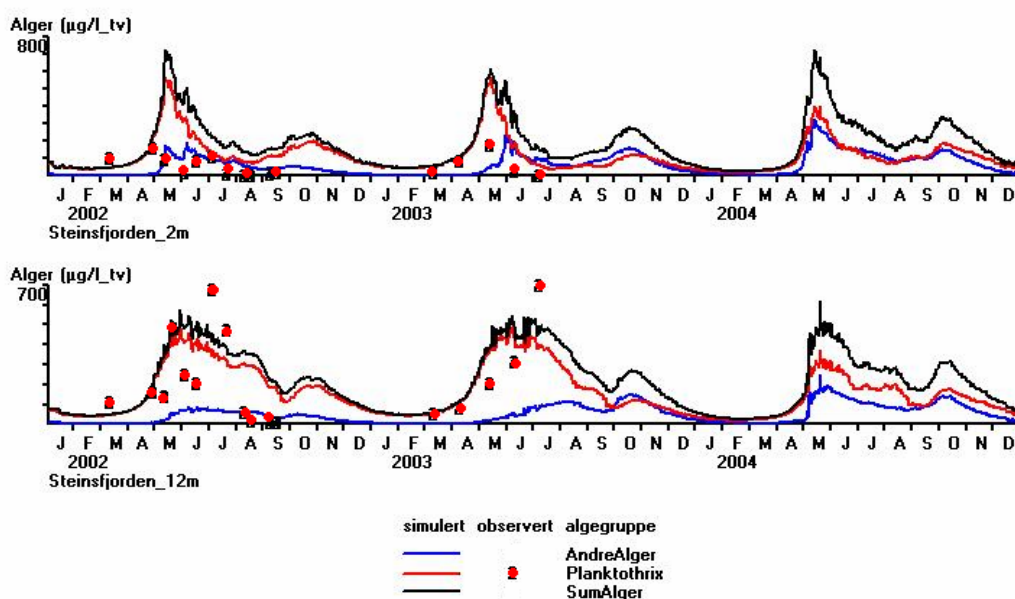
Figur 24. Simuleringene viste i store trekk samsvar med observerte verdier av blågrønnalgen Planktothrix i 2 m og 12 m nivået. I følge observasjonene burde verdiene steget raskere og til større verdier på sommeren, for dermed å falle raskt ned igjen, se 2002-12m. Modellen ga en mer utjevnet fordeling. Den totale algeveksten i løpet av sommeren synes å være omtrent lik. Tolv meter nivået er valgt for å representere maksimumsverdiene i dybdeprofilen. Selv om de simulerte verdiene i blant avviker en del, kan "riktige" verdier finnes ved å sammenlikne med observerte verdier i for eksempel 10 eller 14 meters nivået. Det viktigste er at det totale algeinnholdet i dybdeprofilen er tilfredsstillende for en lengre periode. I 2 meters nivået simulert Planktothrix oppløst om våren for høyt.
