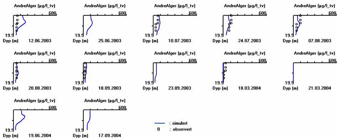
Figur 27. Dybdeprofiler av andre alger (ikke Planktothrix ) sammenliknet med observerte blandprøveverdier.
