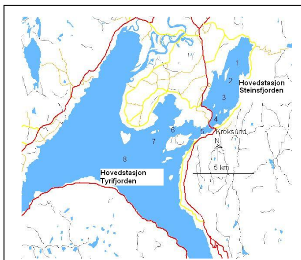
Figur 7. Stasjoner for utskrift av scenariumresultater.
