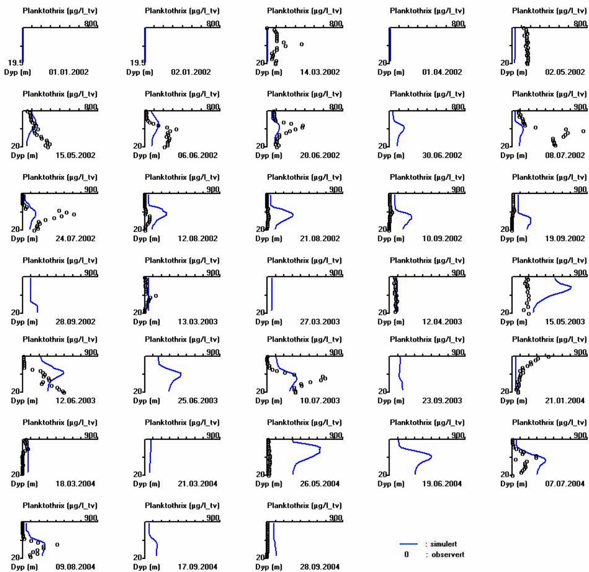
Figur 28. Dybdeprofiler av Planktothrix .
