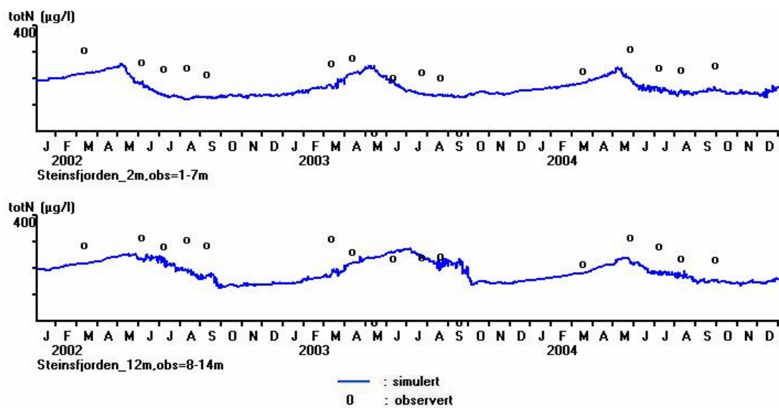
Figur 19. Det var overveiende godt samsvar eller noe lavere simulerte verdier i forhold til observerte verdier av total nitrogen. Nitrogenkonsentrasjonene var vanligvis under 300 \mu\text{g/l} .
