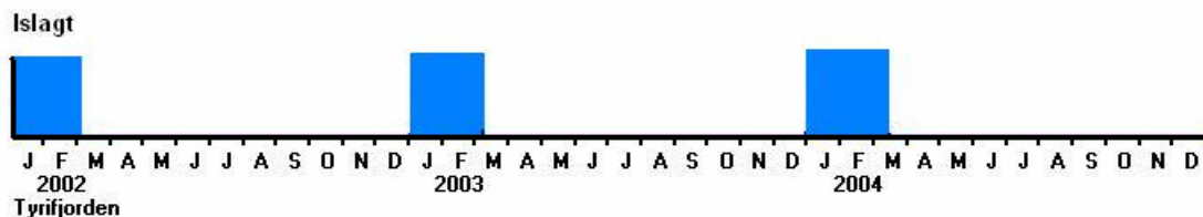
Figur 29. Tyrifjorden ble i følge simuleringene islagt i desember-januar og isfri mars.
