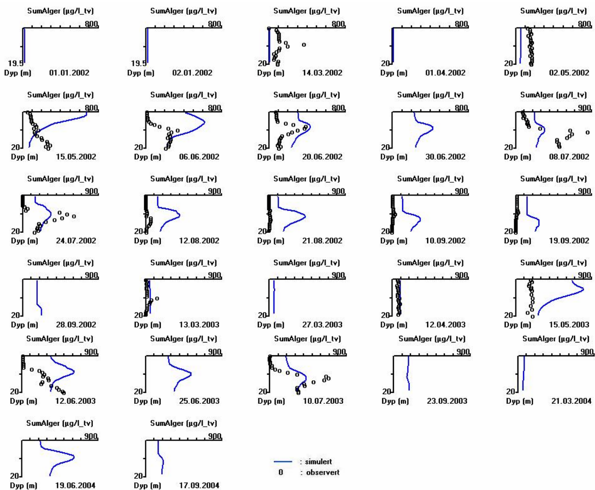
Figur 26. Dybdeprofiler av totalt algeinnhold oppgitt som tørrvekt.
