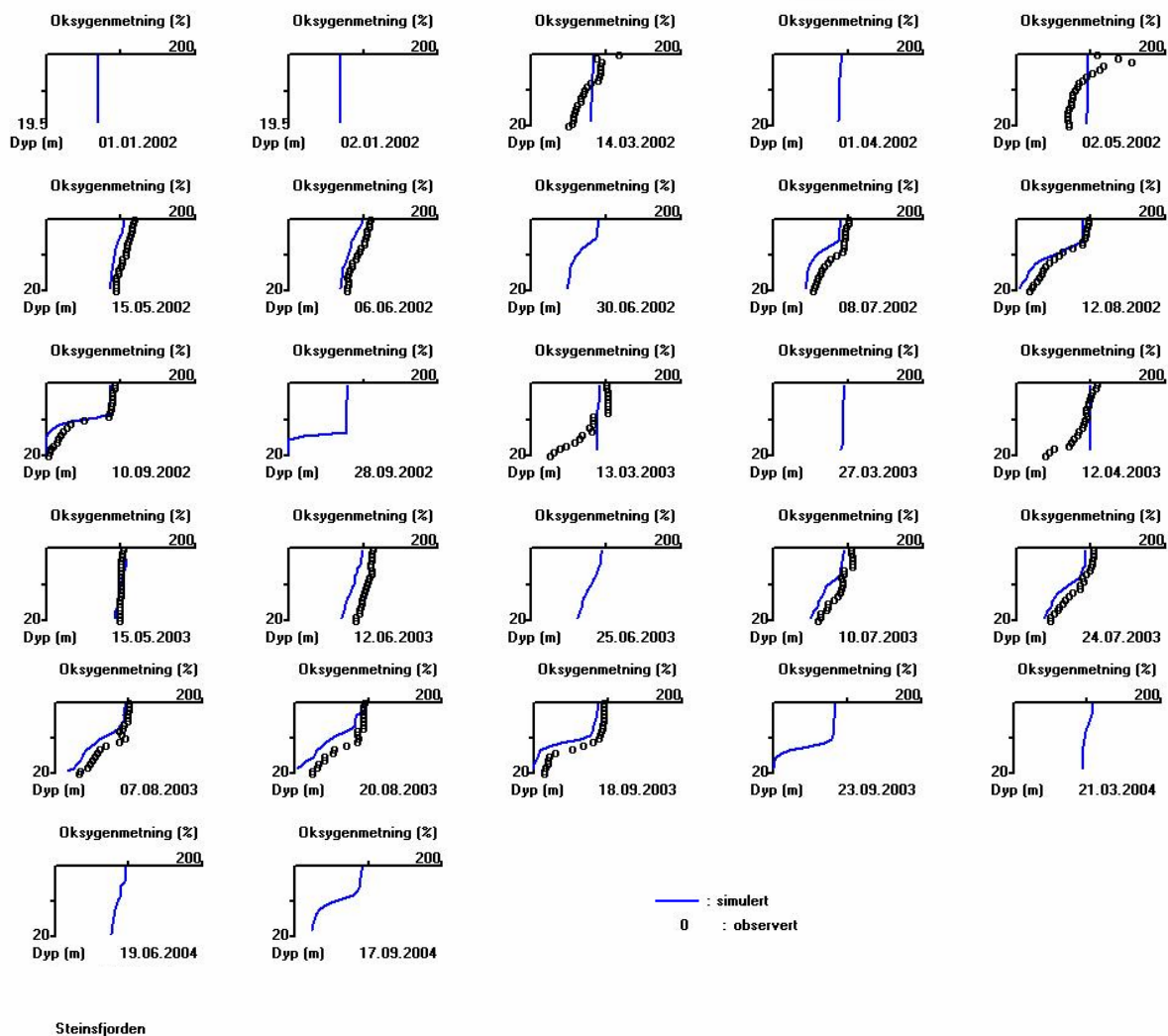
Figur 16. Det var godt samsvar mellom simulert og observert oksygenmetning. Ved oksygensvinn frigir sedimentene næringssalter til vannmassene. Dette var vanlig på sensommeren (august-oktober).
