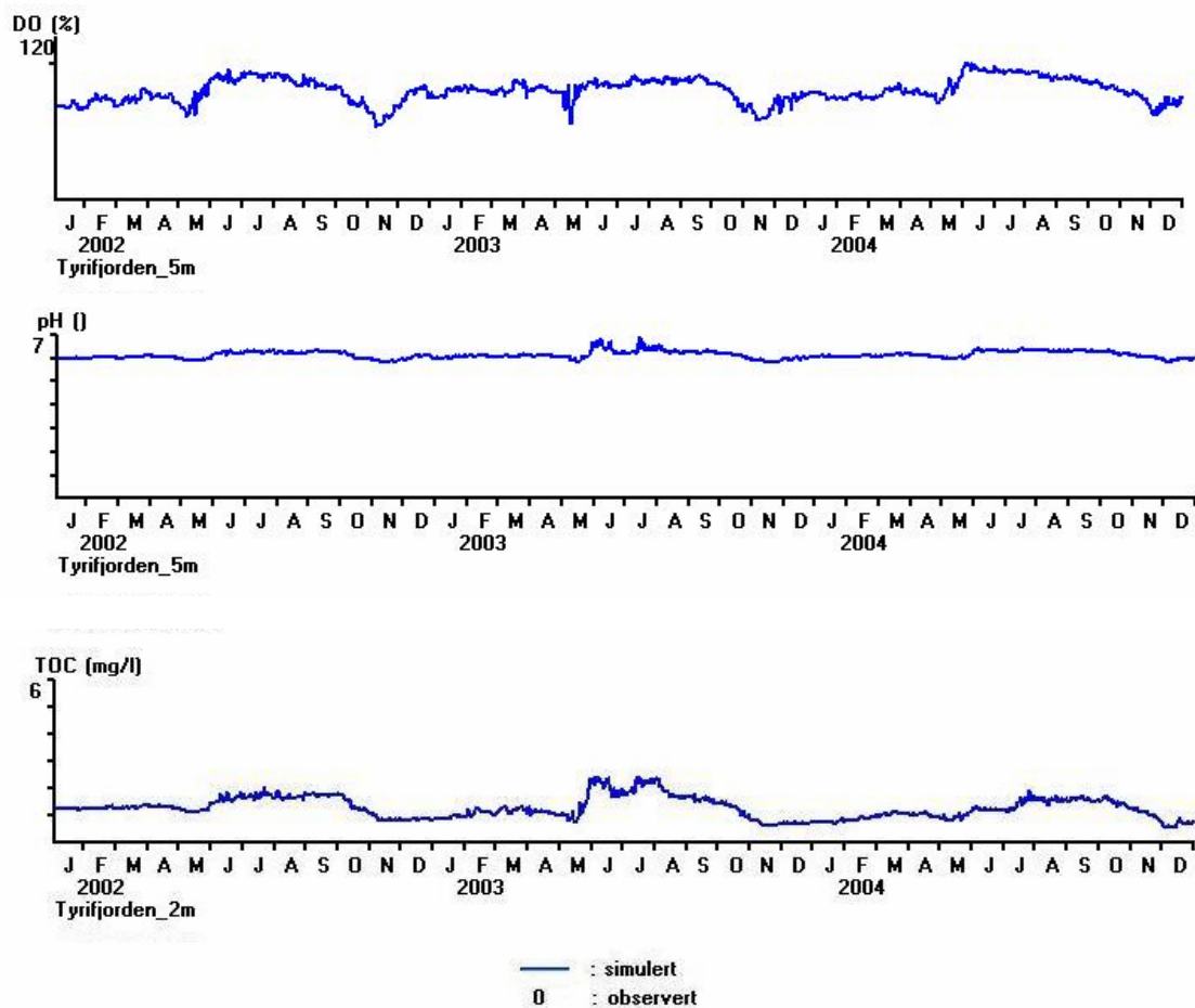
Figur 30. Tyrifjorden. Det var gode oksygenforhold i overflatvannet. PH verdier omkring 6 vitner om gode forhold for eksempel fisk. Totalt organisk karbon var mellom 2 og 4 mg/l.
