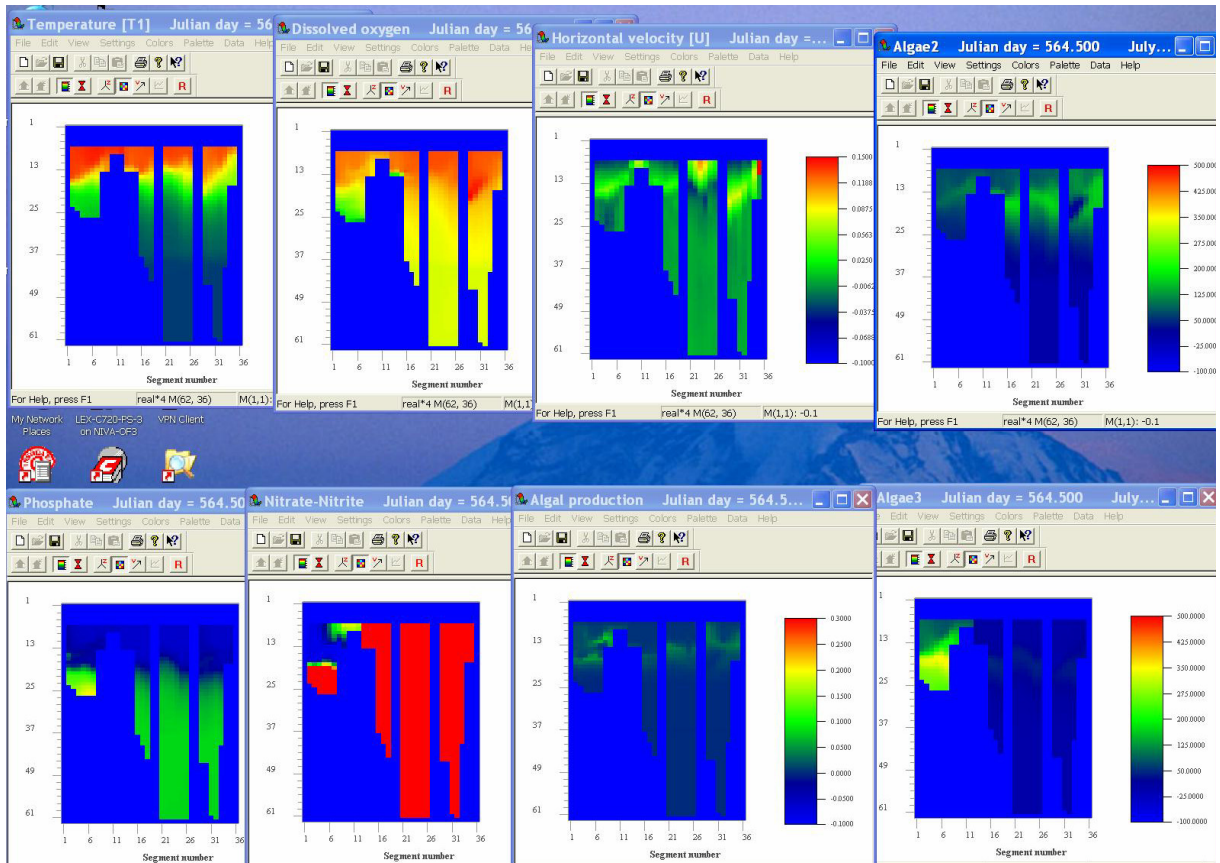
Figur 36. Situasjon i juli 2002, eksempel på indre bølge.
