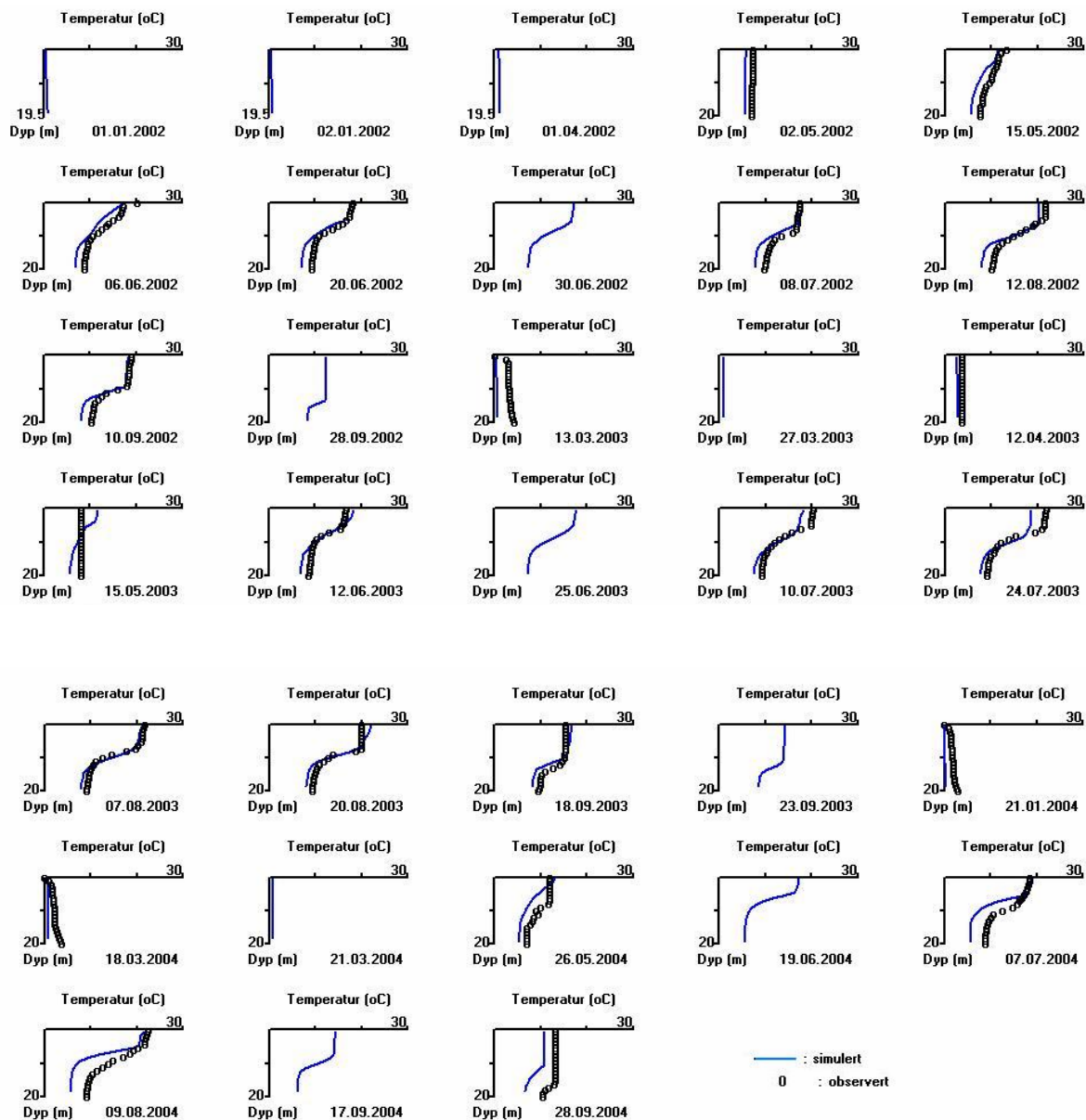
Figur 13. Det var godt samsvar med mellom observerte og simulerte vanntemperaturer. Simuleringene viste til dels noe for kaldt vann nær bunnen.
