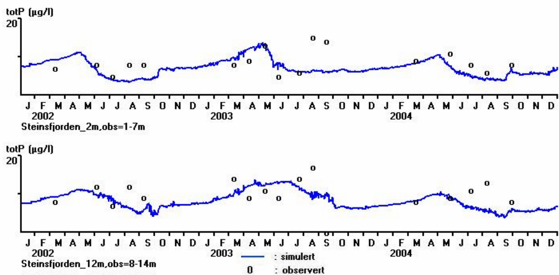
Figur 17. Det var overveiende godt samsvar mellom simulerte og observerte verdier av total fosfor. Verdier omkring 10 \mu\text{g/l} (vannkvalitetsklasse 2) vitner om moderat påvirkning.
