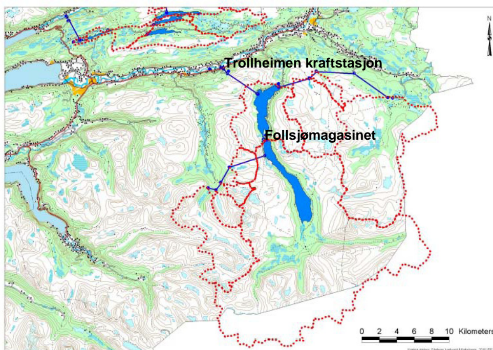
Figur 3: Oversiktskisse av Surnautbyggingen med reguleringsmagasinet Follsjøen (Statkraft, 2005). Et nytt aggregat gir høyere effekt, det gir mindre risiko for driftsavbrudd og stenging, redusert risiko for store vannstandsendringer nedstrøms kraftstasjonen. Endring av inntaket fra bunnvann til overflatevann (flytende system) og endret manøvrering gir bedre levetilstand for laks.
