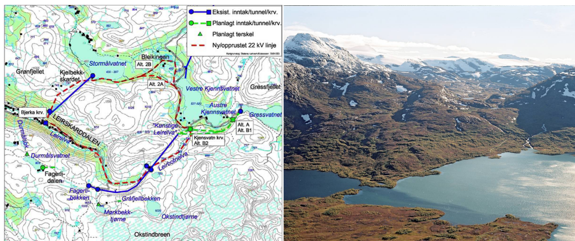
Figur 7: Kartskisse (og bilde) av prosjektet Kjennsvatn, Hemnes kommune Nordland (Statkraft, 2005). Tiltaket vil gi tidlig oppfylling av Gressvatn magasinet, mer stabil vannstand i gressvatn og Kjennsvatna, bedre isforhold, bevegelsesmuligheter for rein, mm.. Dette gir også bedret opplevelsesverdi og tilgjengelighet for friluftslivsinteressene. NVE anbefaler konsesjon alternativ B2. (NVE des. 2005)
