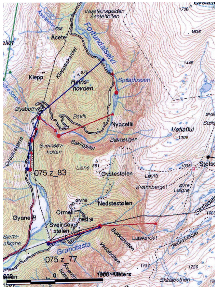
Figur 12: Oversiktskisse av prosjektene i Fortundalselva, fem småkraftverk versus et stort. Røde punkter og linjer viser plassering av småkraftverk, mens blå strek viser mulig overføring for et større anlegg. Samme lengde med elvestreng påvirkes med unntak av noen korte strekk.
