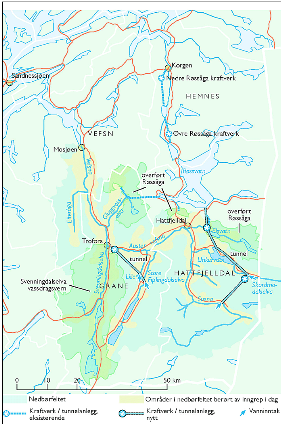
Figur 1: Utbyggingsforslagene i Vefsnas nedslagsfelt. Kilde: Statkraft
