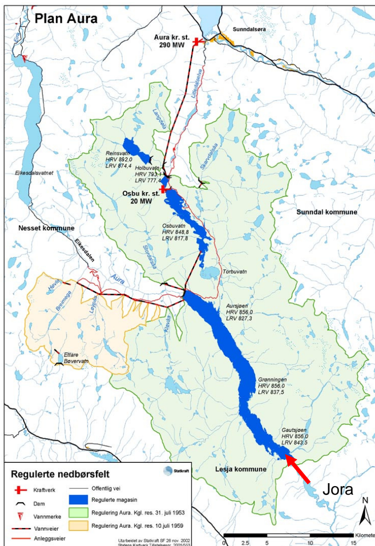
Figur 8: Oversiktskisse av Aurautbyggingen med reguleringsmagasinet Aursjøen (Statkraft, nov. 2002). Tilførsel av nytt vann til Aursjømagasinet kan tenkes overført fra Jora (rød pil). Kilde: Statkraft.
