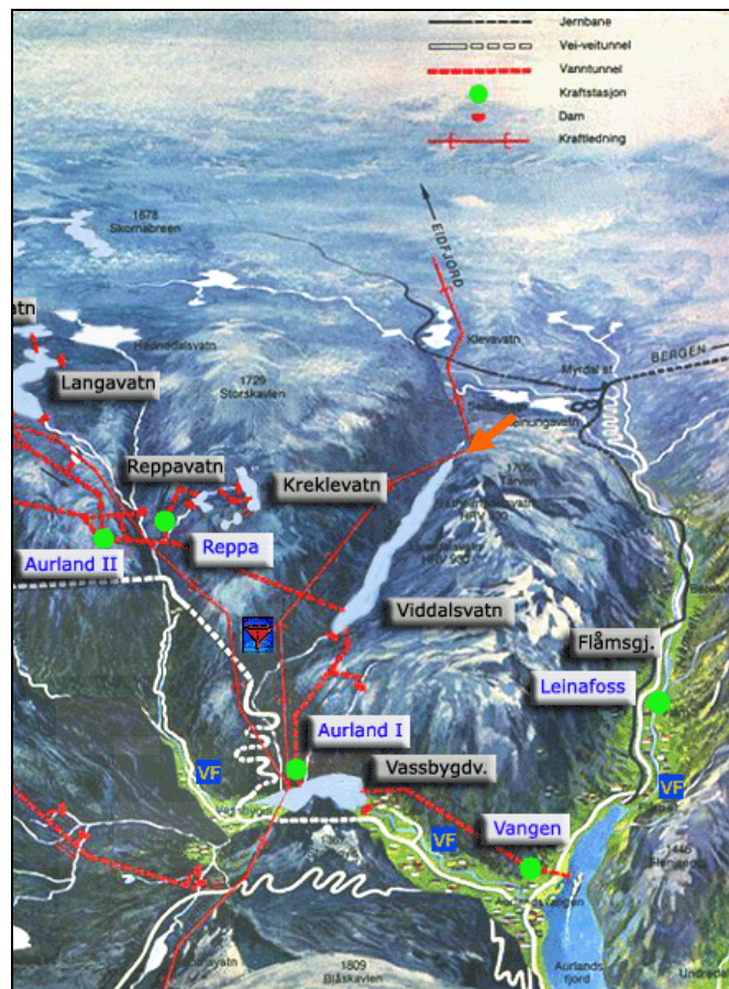
Figur 9: Oversiktskisse av Aurlandutbyggingen (E-CO vannkraft 2005). Mulig tilførsel av vann til Viddalsvatn vist ved bred pil, gir større fleksibilitet i manøvrering av Aurland I og Vangen kraftstasjoner slik at vannføring og temperaturer i Vassbygdvassdraget kan justeres til beste for laksen. Kilde: E-CO Vannkraft
