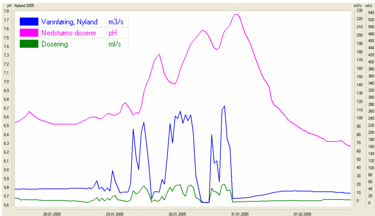
Figur 15. Isstuing oppstrøms Nyland-anlegget førte til overestimering av vannføring og for høy dosering mot slutten av januar 2005. Reaksjonen på pH nedstrøms anlegget (Oksenstein) er vist i figuren. Den reelle vannføringen er sannsynligvis under 20 m 3 /s gjennom hele perioden
