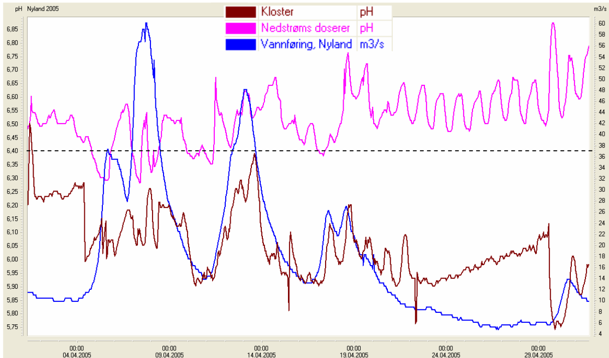
Figur 14. Data fra april 2005 viser at pH-kravet nedstrøms Nyland var satt for lavt til å oppnå pH-målet på 6,4 ved Kloster (stiplet linje). Vannføingen varierte fra 5 til 60 m 3 /s i den aktuelle perioden.
