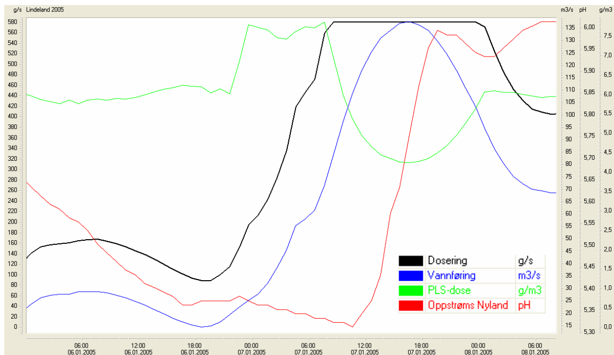
Figur 7. PLS-dosen ble økt i forkant av en kraftig flom 7. januar 2005. Anlegget oversteg maksimal doseringskapasitet i 18 timer, men dosen var likevel så høy at pH oppstrøms Nyland steg fra 5,3 til nærmere 6,0. Transporttiden for vannet mellom Lindeland og Nyland var omkring 11 timer ved dette tilfellet.
