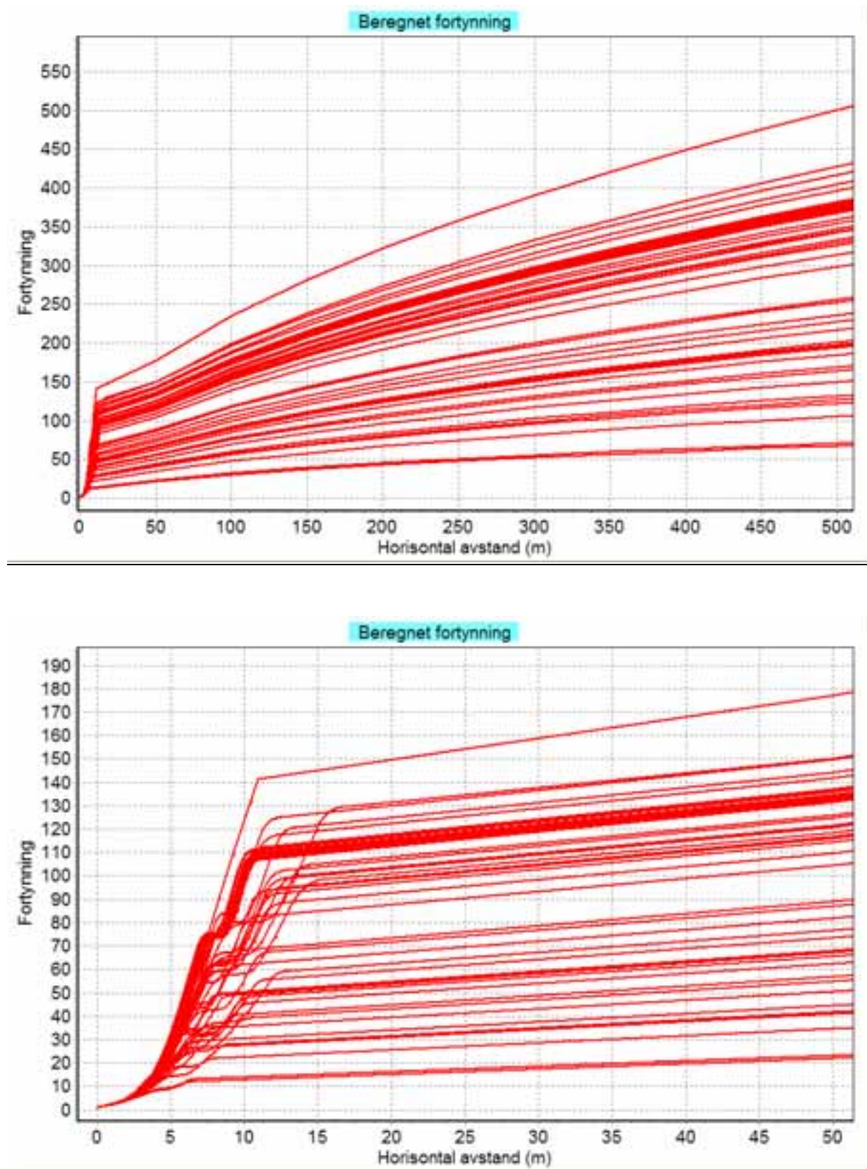
Figur 10. Beregnet fortynning av avløpsvannet for de 50 situasjonene og ved strømhastighet 3 cm/s. Mens den øvre figuren viser resultatet for 0-500 m viser nedre figur 0-50 m.
