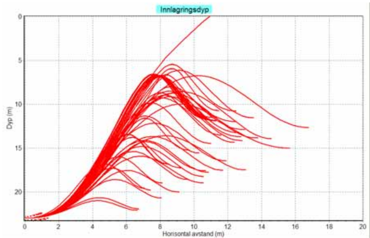
Figur 9. Beregningen av innlagingsdyp for utslippsvannet ved utlipp i 23 m dyp.
