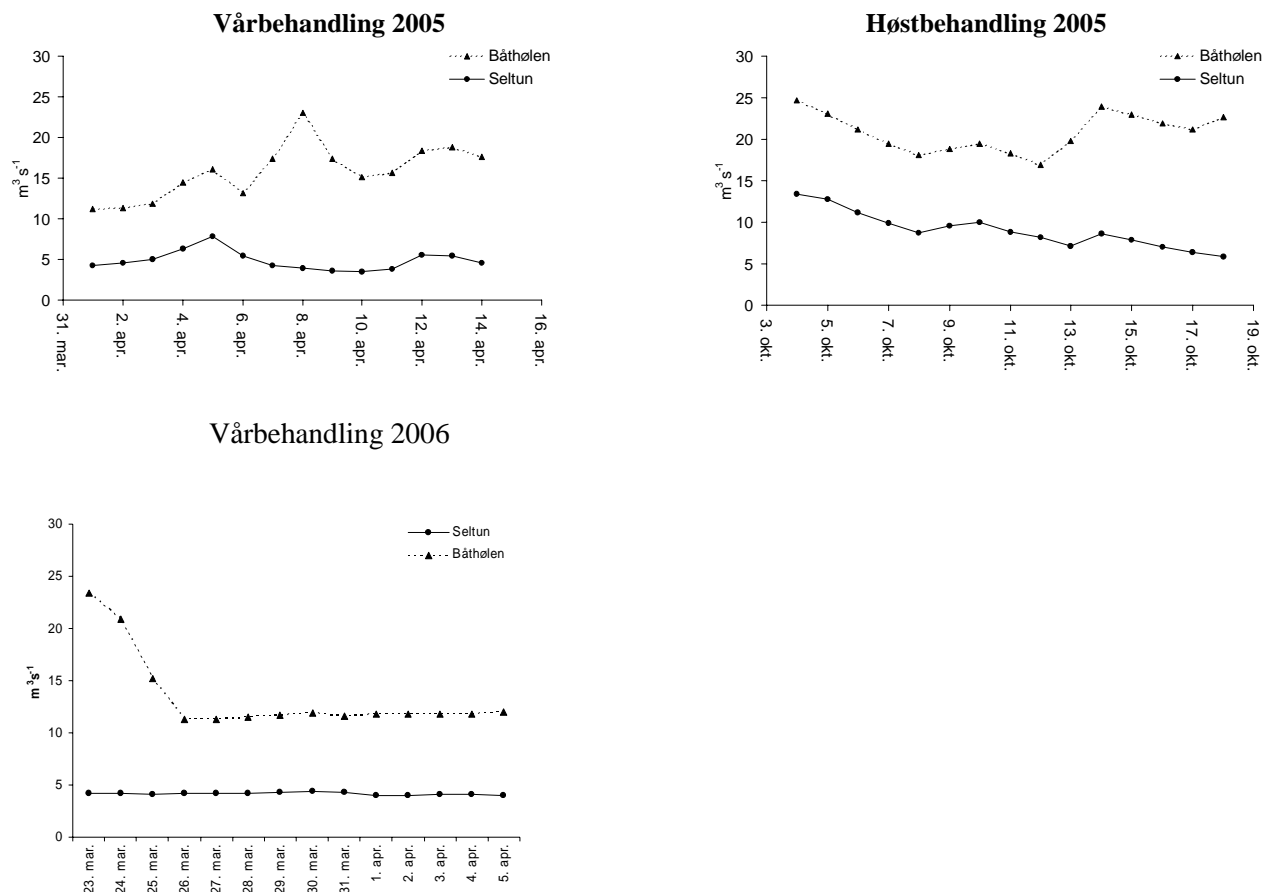
Figur 2 Vannføring ved Seltun (øvre del av behandlet elvestrekning) og Båthølen (nedre del av behandlet elvestrekning) under vår- og høst-behandlingene i 2005 og under vårbehandlingene 2006.
