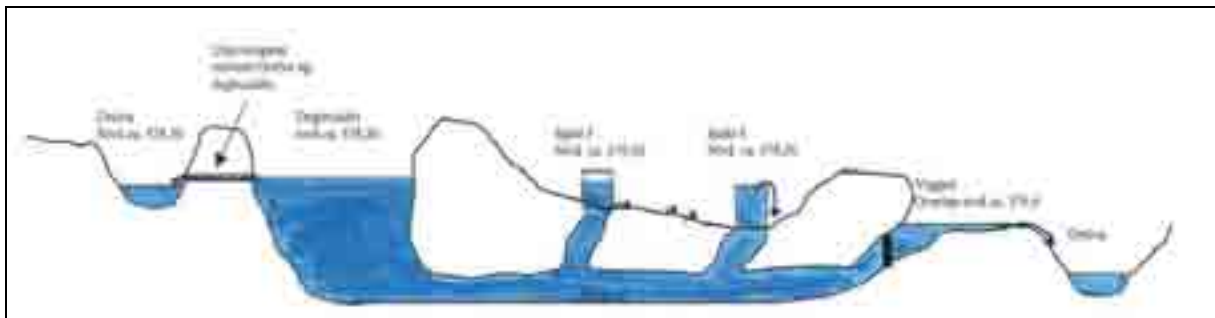
Figur 2. Prinsippskisse, snitt gjennom Orelva, dagbruddet, sjakt 5, sjakt 4 og rampen (veggen) med overløp til Orelva (fra notat av Kjell Kristiansen, Multiconsult, 11.august 2005).
