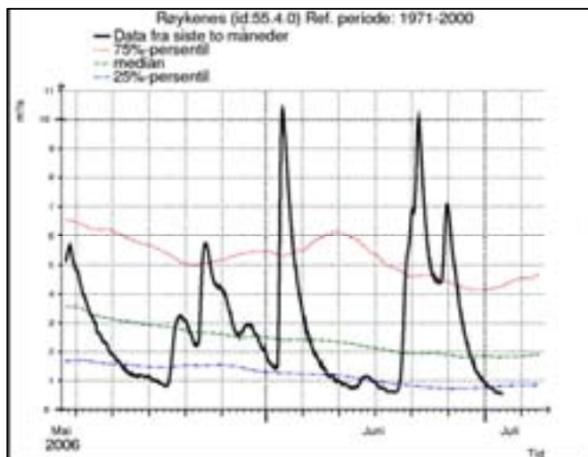
Figur 3. Vannføring ( m^3/s ) registrert i Oselva ved Røykenes i mai-juni 2006. Figuren er hentet fra NVE ( http://www.nve.no ).
