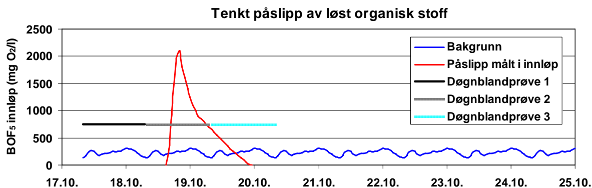
Figur 4.3. Et tenkt påslipp av løst lett nedbrytelig organisk stoff angitt som BOF_5 i innløpet til et rensanlegg. Tidsrom for uttak av tre døgnblandprøver er anvist.
