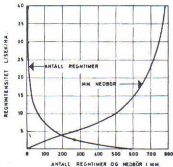
FIG. 10.3. VARIGHETSKURVE FOR INTENSITETEN, OG DE FORSKJELIGE INTENSITETERS BIDRAG TIL DEN SAMLEDE ARSNEDBØR. PLUVIOGRAFMALINGER PÅ BRYNE, TIME KOMMUNE I TIDEN 26-6-65 - 20-6-66.
