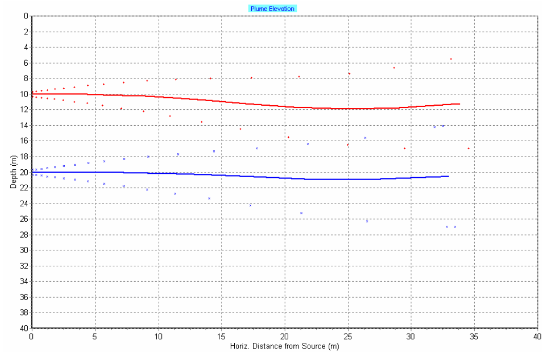
Figur 5. Beregnet bane for utslippssky av kjølevann ved 10 m (rød) og 20 m (blå) utslippsdyp. Beregningene er gjort for sommersituasjon med hydrografidata fra 11. juni 1988. Kryssene viser plumens grenser. Inntaksdyp er 36 m.
