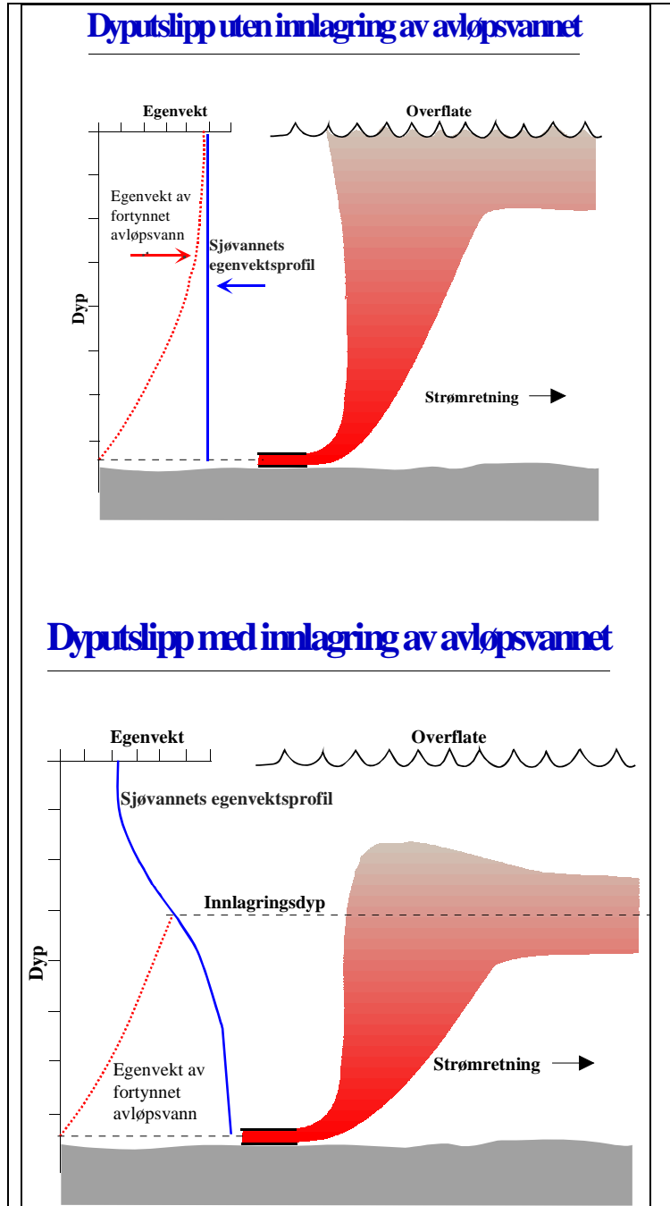
Figur 4. Prinsippkisser som viser hvordan dype utslipp fungerer i forhold til innlagring. En forutsetning for innlagring er at egenvekten for fjordvannet øker med dypet. Ved den øvre figuren er ikke dette tilfelle og utslippsvannet når overflata. I den nedre figuren innlagres utslippet.
