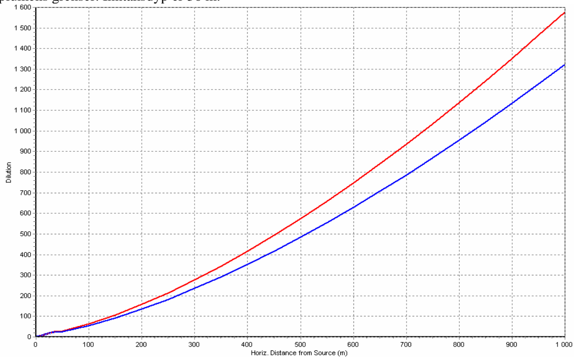
Figur 6. Beregnet fortyning av kjølevann som funksjon av avstand fra utslippspunktet i Saudafjorden ved 10 m (rød) og 20 m (blå) utslippsdyp. Beregningene er gjort for sommersituasjon med hydrografidata fra 11. juni 1988. Inntaksdyp er 36 m.
