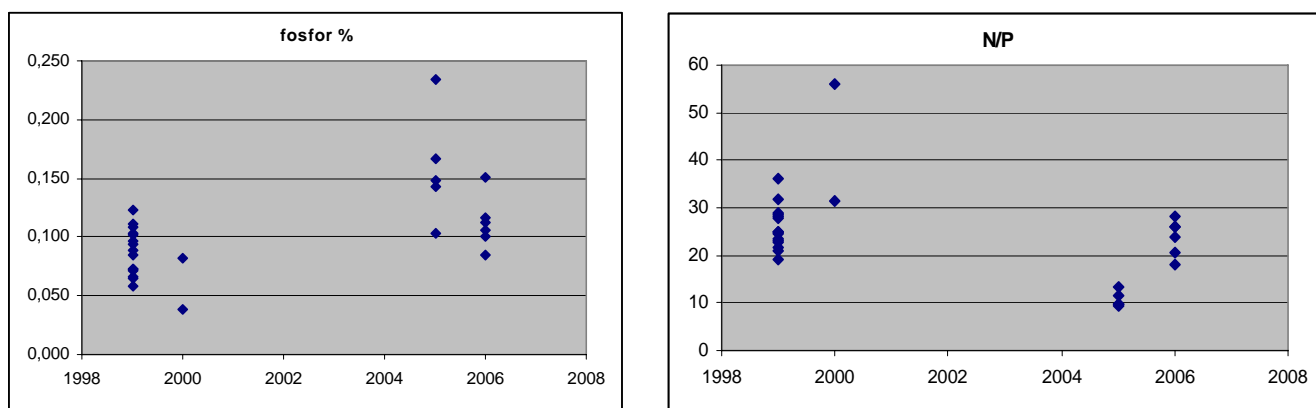
Figur 8. Elementinnholdet i bulk-prøver fra Nedre Lundetjenn i perioden 1998-2006.
