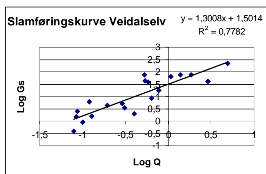
Figur 20 Slamføringskurver for de fire elvene. Q er vannføring; G_s er sedimenttransport. Ligninger gitt i tabell 4.
