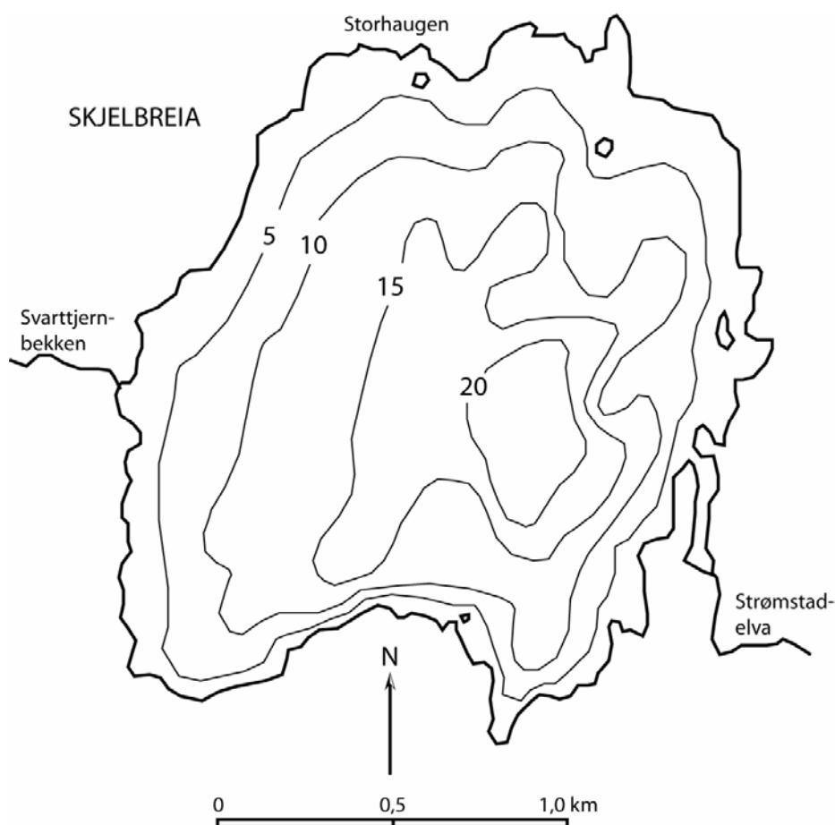
Figur 6. Dybdekart over Skjelbreia. Opploddet av J.E. Løvik, V. Arnesen, J.I. Nordheim og S. Rognerud 2006. 97 målepunkter.
