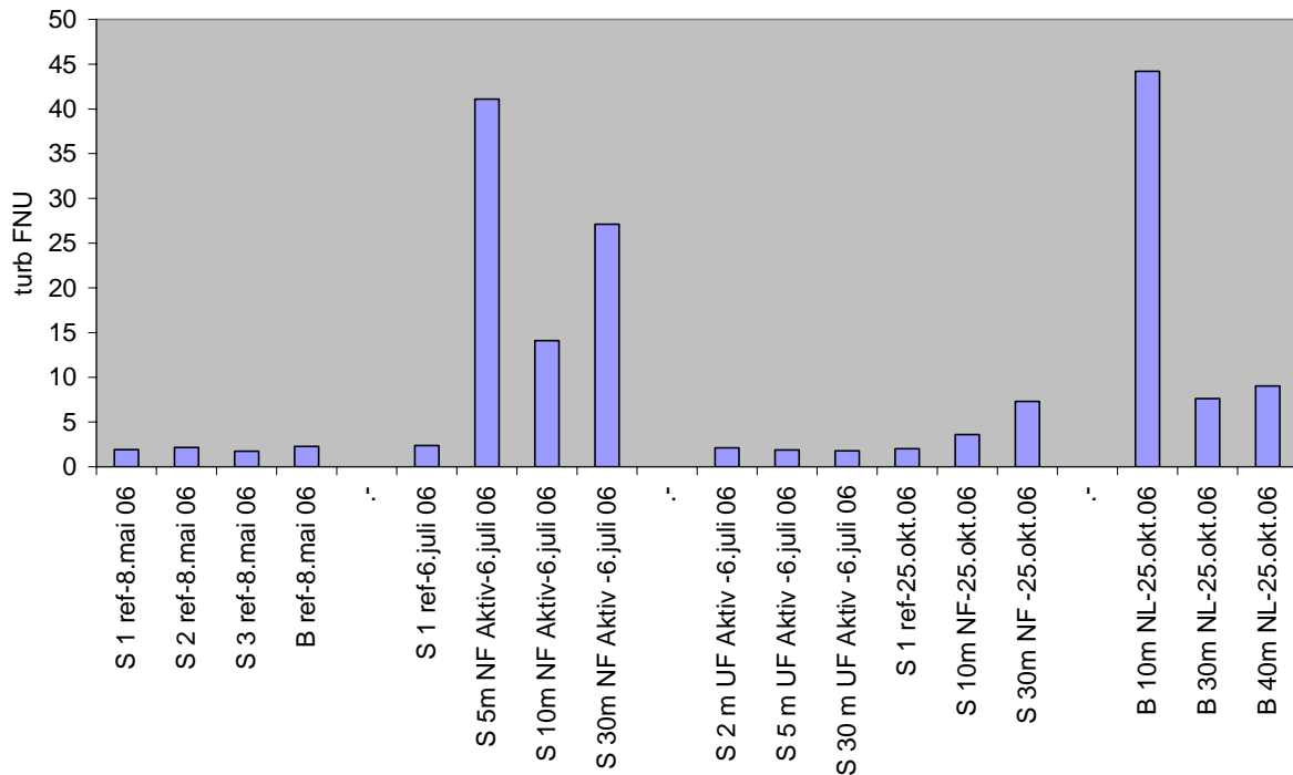
Figur 3. Turbiditet (partikler) i blandprøver fra referansestasjoner og nedstrøms utfylling av tunnelmasser på Strømsøsiden (S) og Bragernessiden (B). Prøvene er tatt i løpet av våren, sommeren og høsten 2006. NF angir nedstrøms fylling, UF angir utover i elva ved fylling, Aktiv angir at prøvene er tatt under aktivt utfyllingsarbeid. Meterangivelse angir avstand fra fylling.
