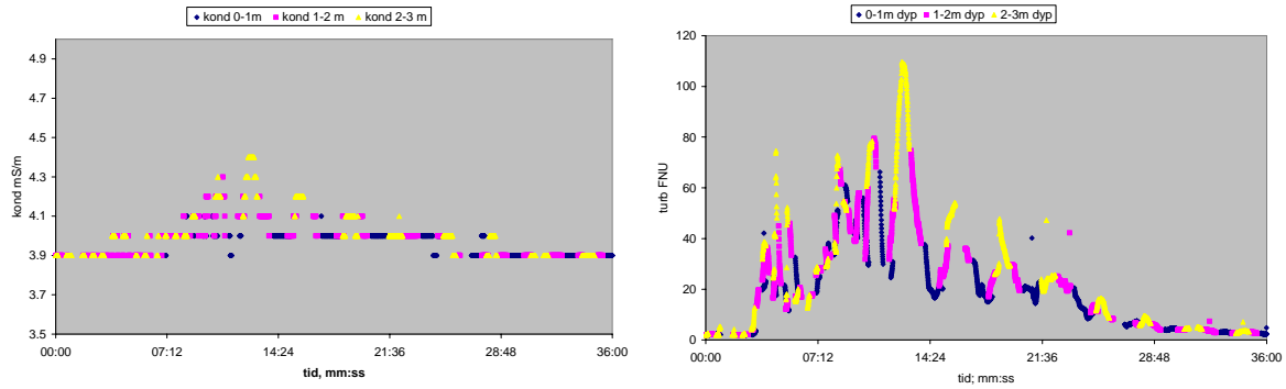
Figur 8. Konduktivitet og turbiditet målt kontinuerlig gjennom ulike dyp 30 m nedstrøms lekker i løpet av deponering av et lekkerlass tunnelmasse på elvebunnen på Bragernessiden. Dybde kategorier angitt med ulike farger.
