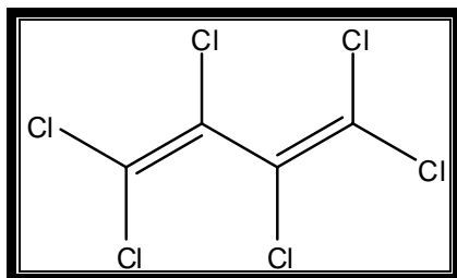
Figur 5. Molekylstrukturen av HCBD
