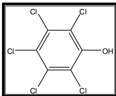
Figur 4. Molekylstrukturen av pentaklorfenol
