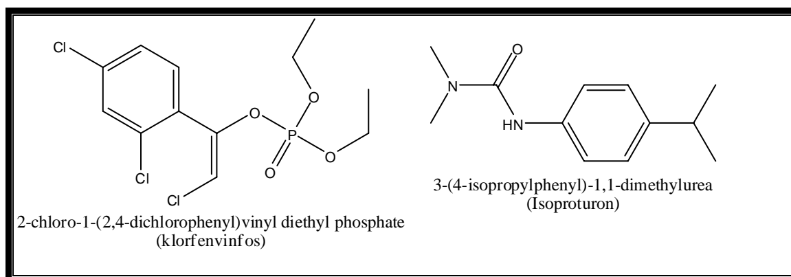
Figur 1. Den kjemiske strukturen til isoproturon og klorfenvinfos.
