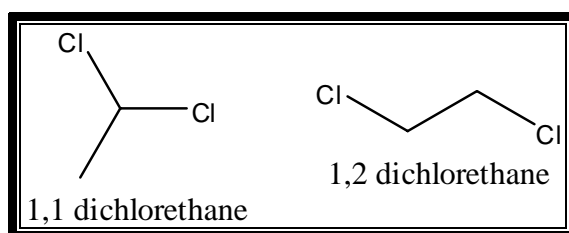
Figur 2. De to mulige molekylstrukturene til dikloretan
