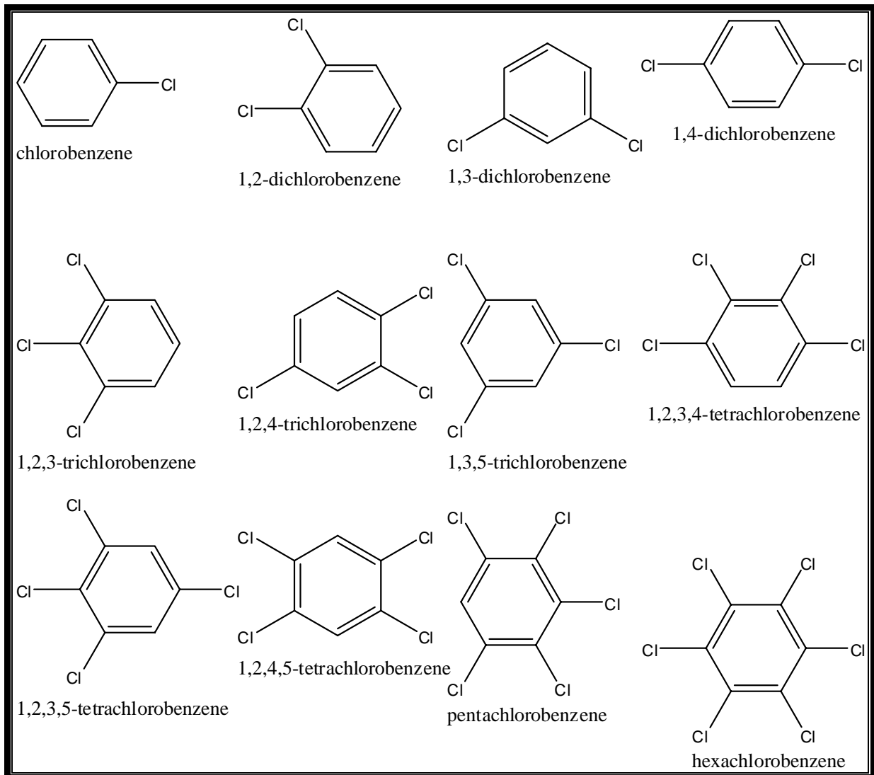
Figur 3. Strukturen til de 12 klorbenzenene
