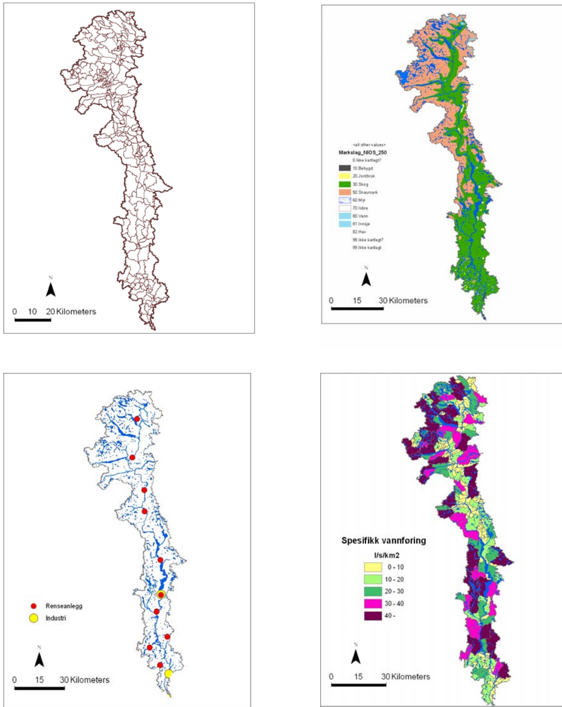
Figur 1. Otras nedbørfelt ble delt inn i NVEs REGINEfelter (320 stk.; øverst, venstre). Tilførsler fra renseanlegg og industri (nedre, venstre) ble i modellen tilført vassdraget innen omsluttende REGINEfelter. Arealtyper (øvre, høyre) for hvert REGINEfelt ble funnet ved bruk av GIS. Det ble beregnet tilførsler fra ulike arealtyper ved å nytte avrenningskoeffisienter og vannføring. Vannføring ble beregnet fra spesifikk avrenning (nedre, høyre) innen hvert REGINEfelt.
