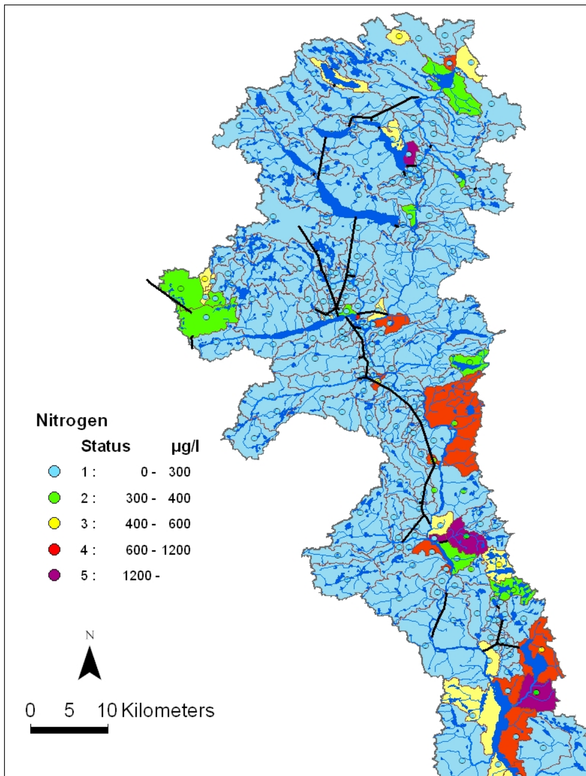
Figur 8. Nitrogenkonsentrasjoner i øvre del av Otra. Bakgrunnsfargen viser lokal konsentrasjon, dvs. tilførsler dividert på vannføring kun innen eget REGINEfelt. Punktene viser midlere konsentrasjoner i elvene. Vannveier for reguleringer er vist med svarte streker.
