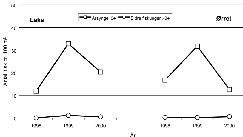
Figur 30. Tetthet (antall pr. 100 m 2 ) av laks- og ørretunger i lakseførende del av Otra i 1998–2000. Data fra Kroglund m.fl. (2000).
