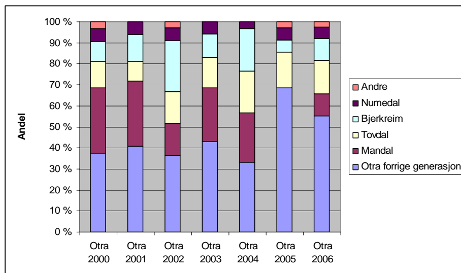
Figur 25. Beregning av den mest sannsynlige tilhørigheten til voksen villaks i Otra i årene 2000 til 2006, ut fra genetisk klassifisering av \geq 30 individer i forhold til mulige kilder. 'Andre' betyr at selv den mest sannsynlige tilhørigheten er sjelden ( < 1/1000 ) i forhold til bestandens genetiske sammensetning, og at disse individene derfor kan komme fra andre kilder.
