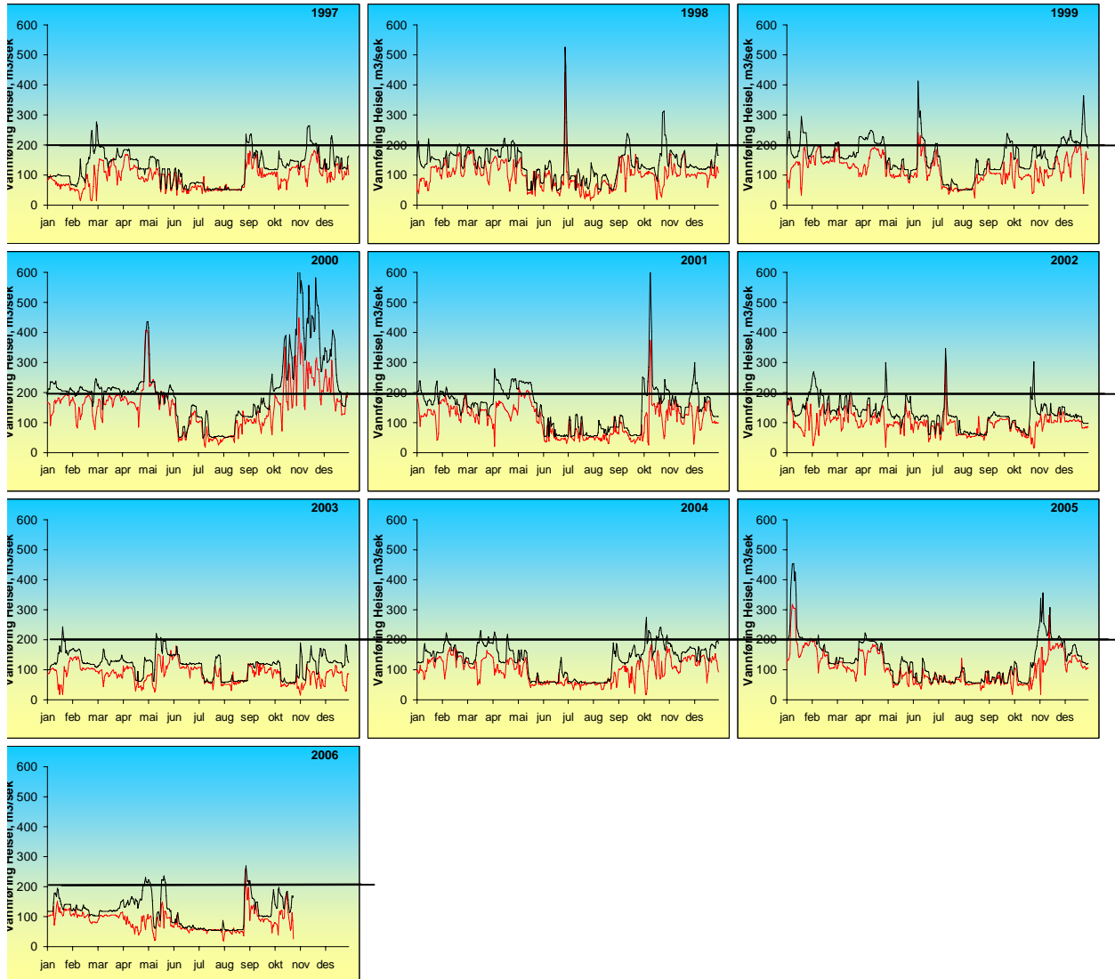
Figur 4. Vannføring ( \text{m}^3 \cdot \text{s}^{-1} ) ved Heisel (sort strek) og ut av Byglandsfjorden (rød strek) for perioden 1997 til 2006. Vannføringer >200 \text{ m}^3 \cdot \text{s}^{-1} er angitt med horisontal sort strek.
