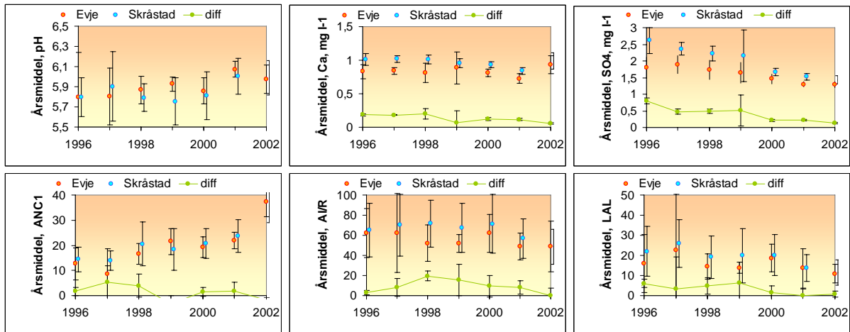
Figur 19. Årsmidler i pH, \text{SO}_4 , Ca, ANC, RAI og LAL ved henholdsvis Evje og Skråstad. Det benyttes kun data fra NIVA i denne analysen. Differanse i middelverdi mellom Evje og Skråstad er beregnet. Vertikale linjer angir \pm 1 standardavvik.
