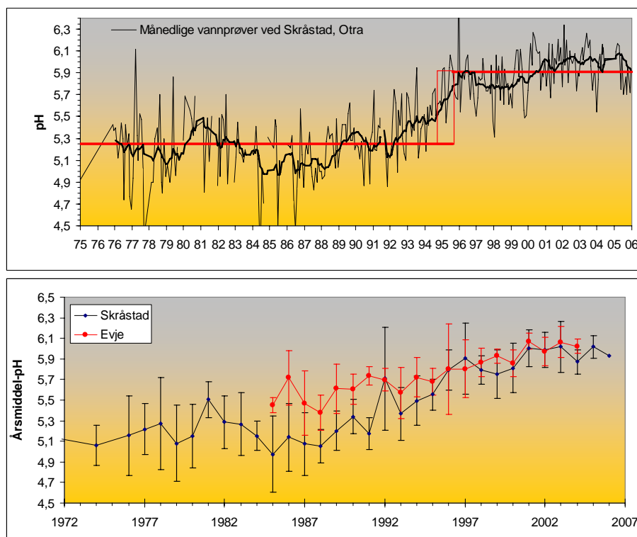
Figur 6. a) Månedlige pH-målinger ved Skråstad (1975–2006). Midlere pH for perioden 1975–1996 og for perioden 1996–2006 er indikert. Rød "boks" antyder igangsetting av industriledningen. b) Årsmiddel pH ( \pm 1 SD) for stasjonene Evje og Skråstad.
