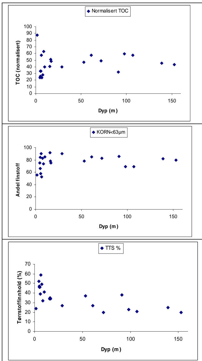
Figur 5. Organisk innhold (TOC normalisert, \mu\text{g}/\text{mg} ), andel finfraksjon (Korn < 63 \mu\text{m} ) og tørrstoffinnhold (TTS %) i overflatesediment som funksjon av bunn dyp på prøvetaksstedet.
