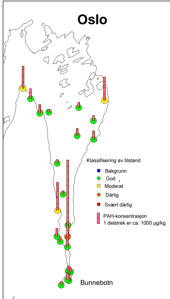
Figur 12. Konsentrasjoner av \Sigma PAH16 i sedimenter på de ulike stasjonene. I figuren er konsentrasjonen på hver stasjon vist som en søyle. Fargen på basis til hver søye tilsvare resultatet av klassifiseringen vist i Tabell 8.
