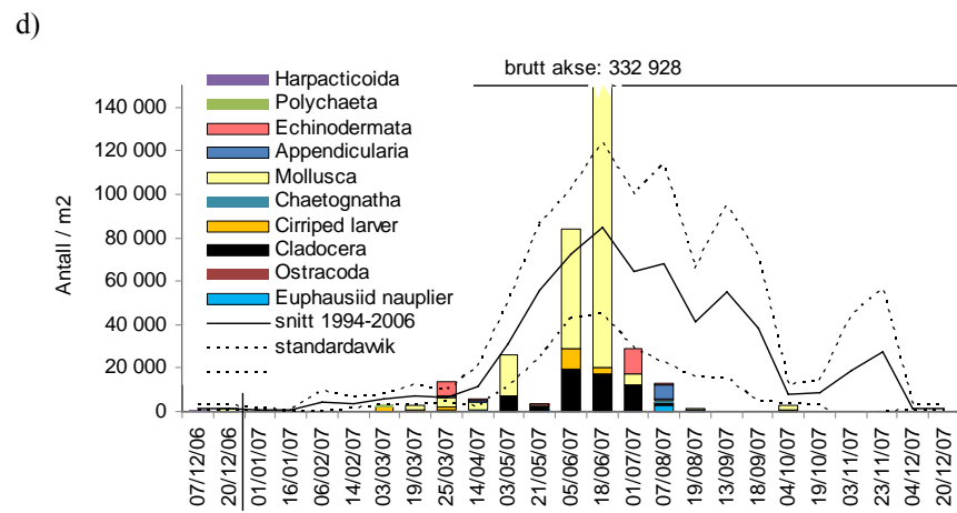
Figur 5.9 Fordeling av dyreplankton i de øvre 50 m i 2007 på Arendal St. 2 fordelt på ulike grupper og på enkelte arter. a) Calanus -stadier, b,c,d) enkeltarter. Gjennomsnitt og standard avvik er vist for perioden 1994-2006 .
