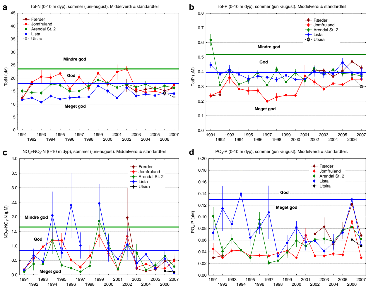
Figur 4.6. Næringsalter i overflatevann (0-10m dyp) sommerstid (juni-august). a) Tot-N, b) Tot-P, c) NO 3 +NO 2 -N og d) PO 4 -P (µM). SFTs klassifiseringsgrenser er markert.
