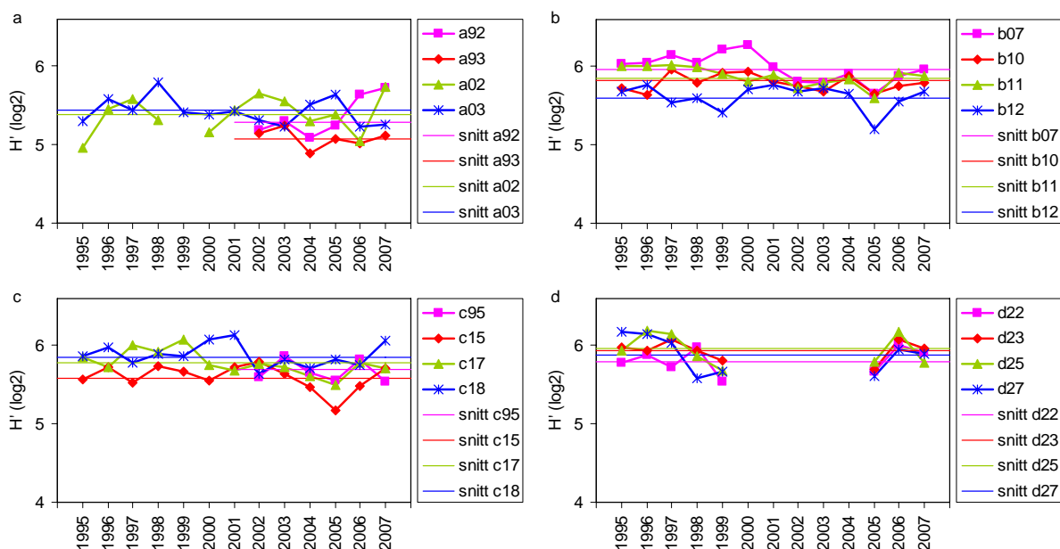
Figur 6.1. Biologisk mangfold i hardbunnssamfunn på gruntvann langs kysten av Sør-Norge i region A, B, C og D. Biomangfold er basert på Shannon indeks H'(\log_2) og forekomst av alger og dyr er gitt som sum over dyppet av e^x hvor x er: 1=enkeltpunkt, 2=sjelden, 3=vanlig, 4=dominerende. Gjennomsnitt er beregnet for perioden 1995 (2002)-2006.
