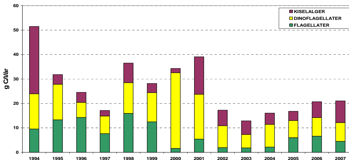
Figur 5.6 Total planteplanktonbiomasse ( \mu\text{g C/l/år} ) integrert over året for perioden 1994-2007.
