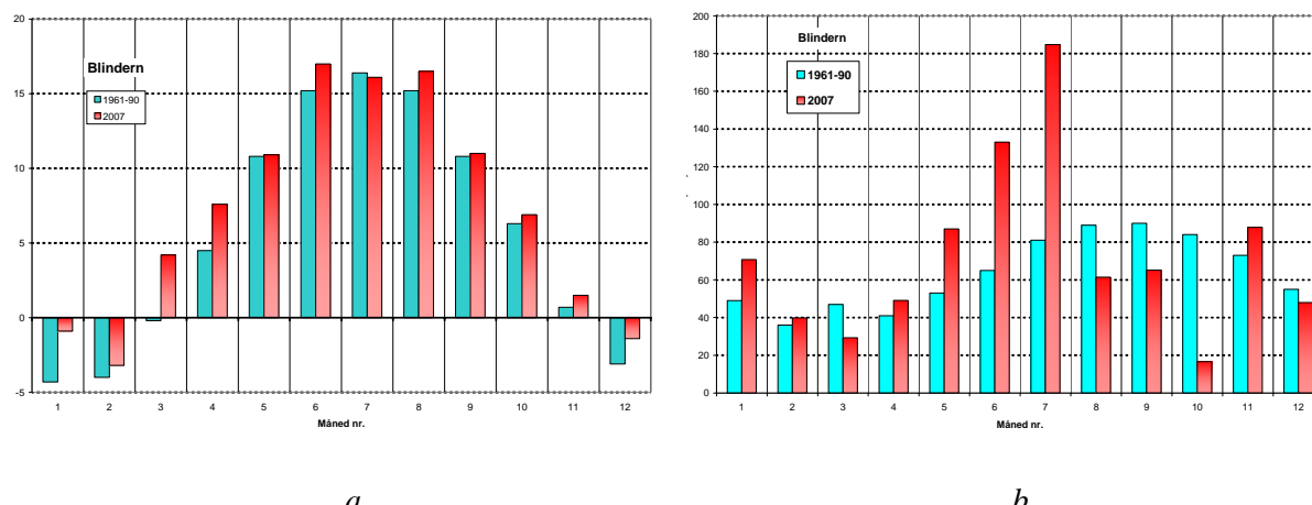
Figur 2.3 Månedsmiddeltemperatur (a) og nedbør (b) ved Blindern (Oslo) i 2007 (røde søyler) sammenlignet med midlere (blå søyler) lufttemperatur og normal nedbør 1961-90. (Data fra Meteorologisk institutt).
