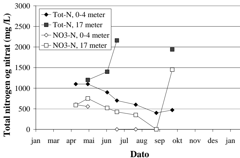
Figur 26. Målte konsentrasjoner av total fosfor, total nitrogen (Tot-N) og nitrat (NO 3 -N) i overflatelaget (0-4 m) og i bunnlaget (17-18 m) i Kolbotnvannet 2007.
