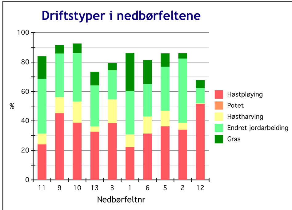
Figur 7: Fordeling av driftsformer i de ulike delnedbørfeltene (%). Delnedbørfeltene er 11 = Leira midtre nord fra Kringler til Krokfoss, 9 = Songa og Vikka, 10 = Tveia og Nordbytjern, 13 = Leira midtre sør fra Krokfoss til Leirsund, 3 = Gjermåa øvre, 1 = Mikkelsbekken, 6 = Ulvedalsbekken, 5 = Gjermåa, 2 = Jeksla, 12 = Leira nedre fra Leirsund til samløp med Nitelva.
