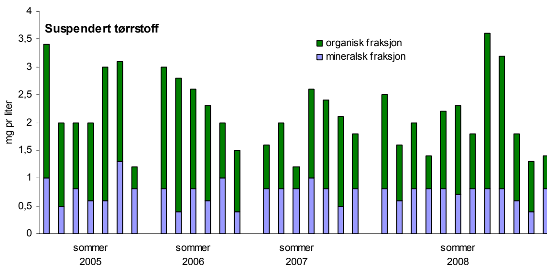
Figur 4. Innholdet av suspendert tørrstoff i vannet (mg/L) i Lyseren vist for de fire årene 2005 - 2008. Fraksjoner av organisk og mineralsk stoff er markert.
