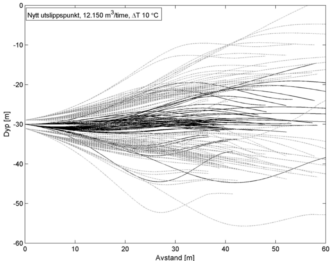
Figur 35. Utslippsplumen fra nytt separat utslipp av kjølevann fra ACC sitt CO 2 -fangstanlegg til 30 m dyp, diameter 2,9 og helningsvinkel 10°. Figuren viser vertikalutstrekning i ulike avstander fra utslippspunktet. Heltrukken svart linje viser senterlinjen mens øvre og nedre utstrekning er vist som grå stiplede linjer. Merk at bunndypet ved utslippspunktet vil være ca 30 m. En synkende utslippssky indikerer derfor at kjølevannet vil følge bunntopografien.
