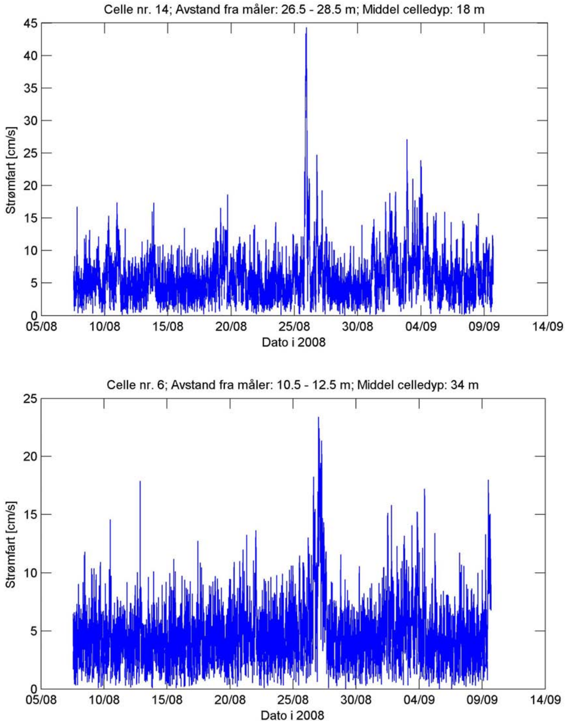
Figur 26. Målt strømhastighet (cm/s) i 18 og 34 m dyp, 2. måleperiode.
