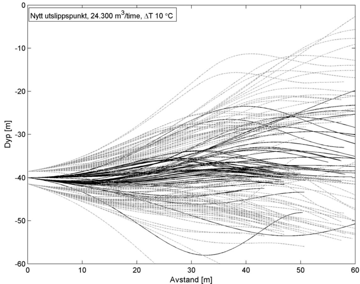
Figur 36. Utslippsplumen fra nytt separat utslipp av kjølevann fra ACC sitt CO 2 -fangstanlegg til 40 m dyp og diameter 2,9. Figuren viser vertikalutstrekning i ulike avstander fra utslippspunktet. Heltrukken svart linje viser senterlinjen mens øvre og nedre utstrekning er vist som grå stiplede linjer. Merk at bunndypet ved utslippspunktet vil være ca 30 m. En synkende utslippssky indikerer derfor at kjølevannet vil følge bunntopografien.
