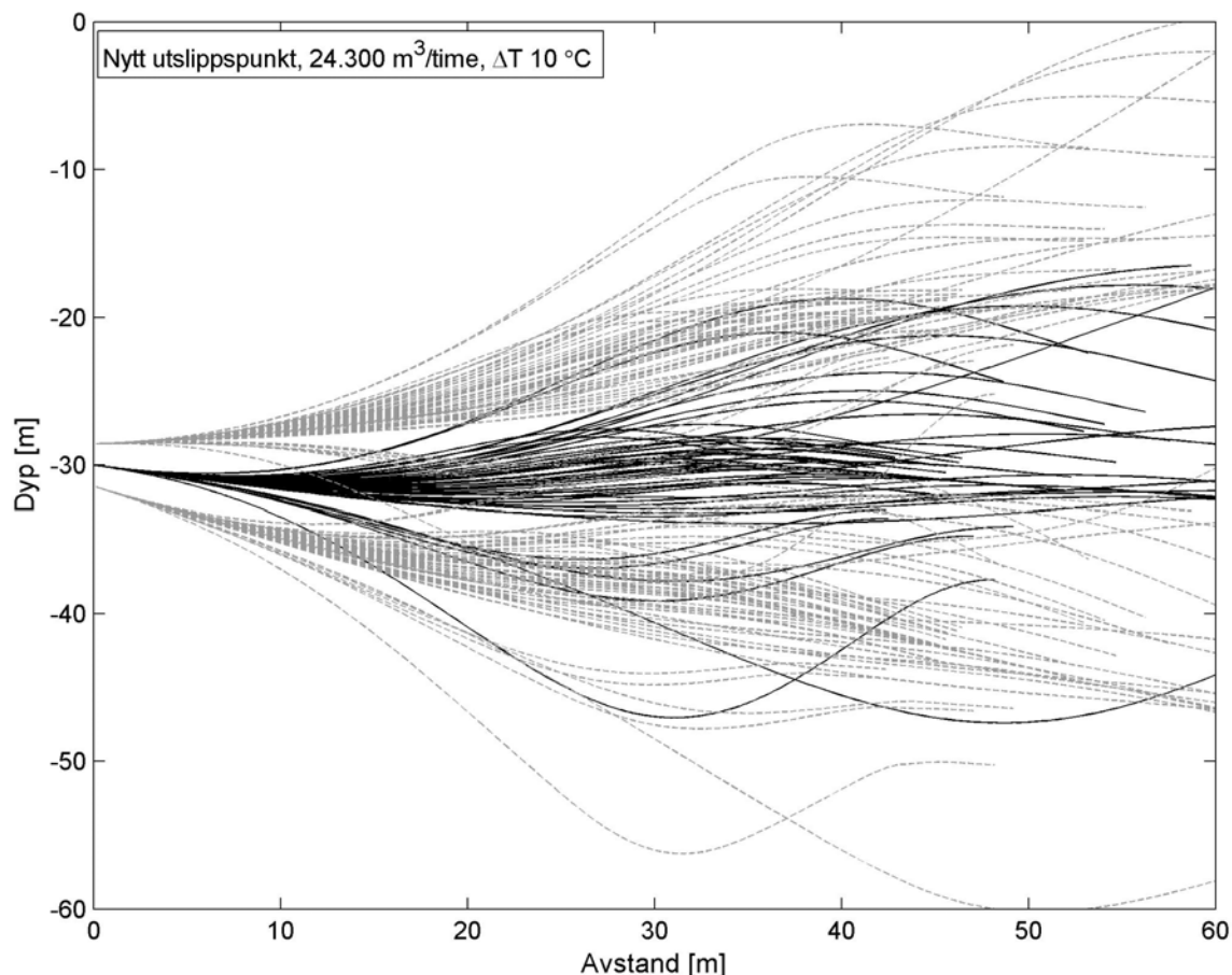
Figur 34. Utslippssplumen fra nytt separat utslipp av kjølevann fra ACC sitt CO 2 -fangstanlegg til 30 m dyp, diameter 2,9 og helningsvinkel 10 °. Figuren viser vertikalutstrekning i ulike avstander fra utslippspunktet. Heltrukken svart linje viser senterlinjen mens øvre og nedre utstrekning er vist som grå stiplede linjer. Merk at bunndypet ved utslippspunktet vil være ca 30 m. En synkende utslippssky indikerer derfor at kjølevannet vil følge bunntopografien.
