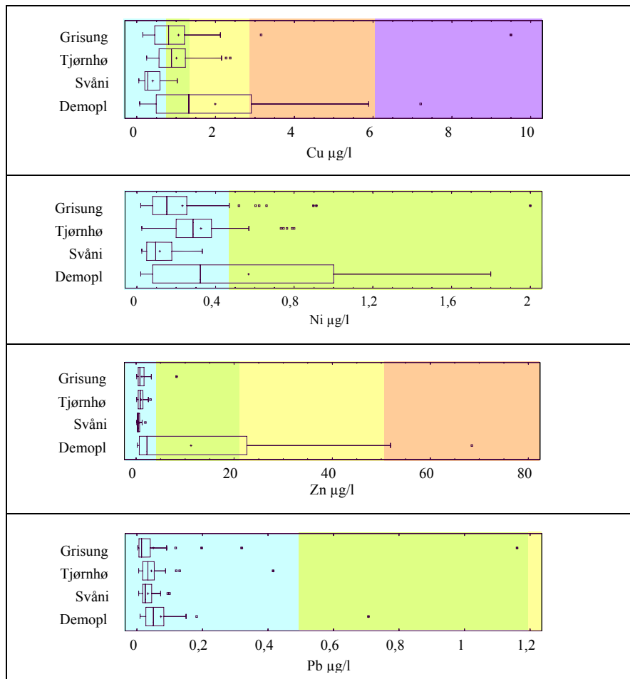
Figur 12. Boksplott for konsentrasjonene av de viktigste metallene i delfeltene (2002 og 2003). Boksene inkluderer 50 % av observasjonene, medianen er markert med strek og middelverdien med +. Linjene fra boksene er trukket til laveste og høyeste kvartil (25 til 75 % av observasjonene), mens observasjoner utenfor disse er markert med firkanter. Fargeangivelsene representerer SFTs tilstandsklasser for metaller i vann. Blå: ubetydelig forurenset, grønn: moderat forurenset, gul: markert forurenset, orange: sterkt forurenset og rød: meget sterkt forurenset.
