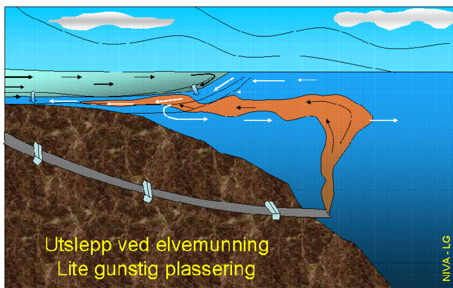
Figur 4. Illustrasjon av utslepp nær ei elvemunning, der kompensasjonsstraumen fører fortynna avlaupsvattn innover (ugunstig arrangement).
