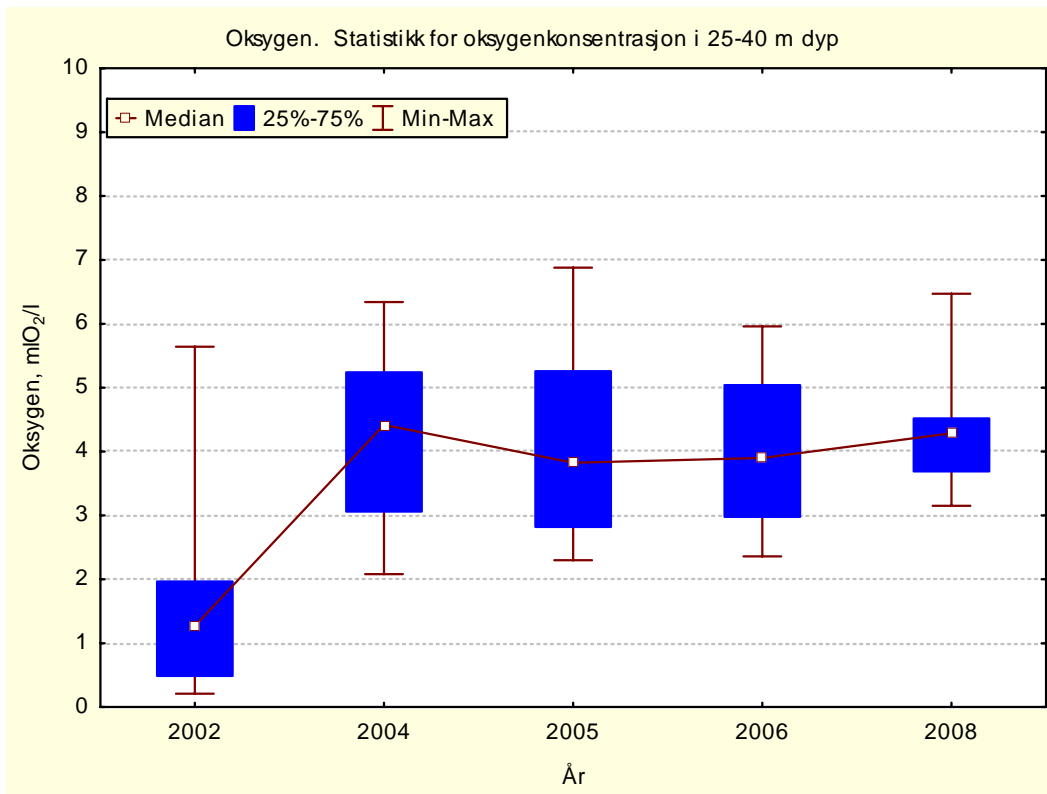
Figur 14. Oppsummerende statistikk for oksygenmålinger ( \text{mlO}_2/\text{l} ) i Havnebassenget (øvre figur, 25-40 m dyp) og ved Lindenes (nedre figur, 25-80 m dyp) i tidsrommet 2002-2008. En stor forbedring kan observeres etter at utslippet fra Odde smelteverk stoppet høsten 2002.
