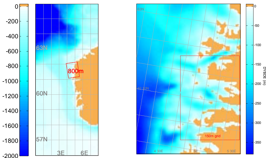
Figur 3. Kart over modell med 4 km oppløsning (venstre) og 800 m oppløsning (høyre).
