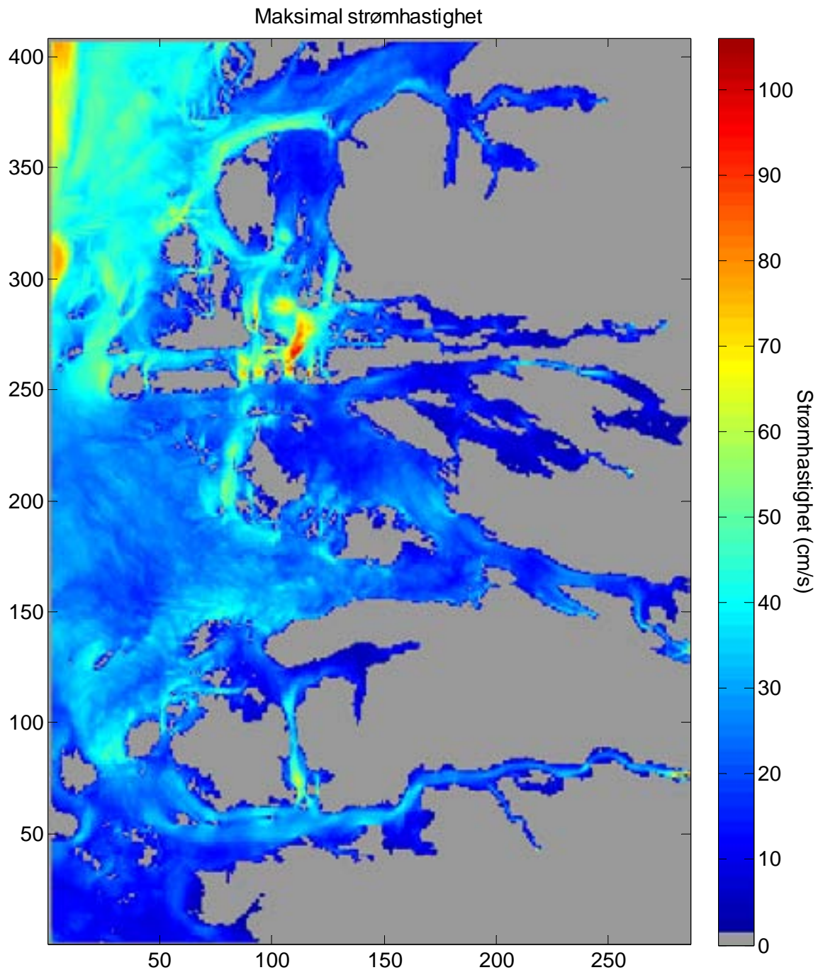
Figur 11. Maksimal strømhastighet i overflatelaget i løpet av en ukes beregninger.
