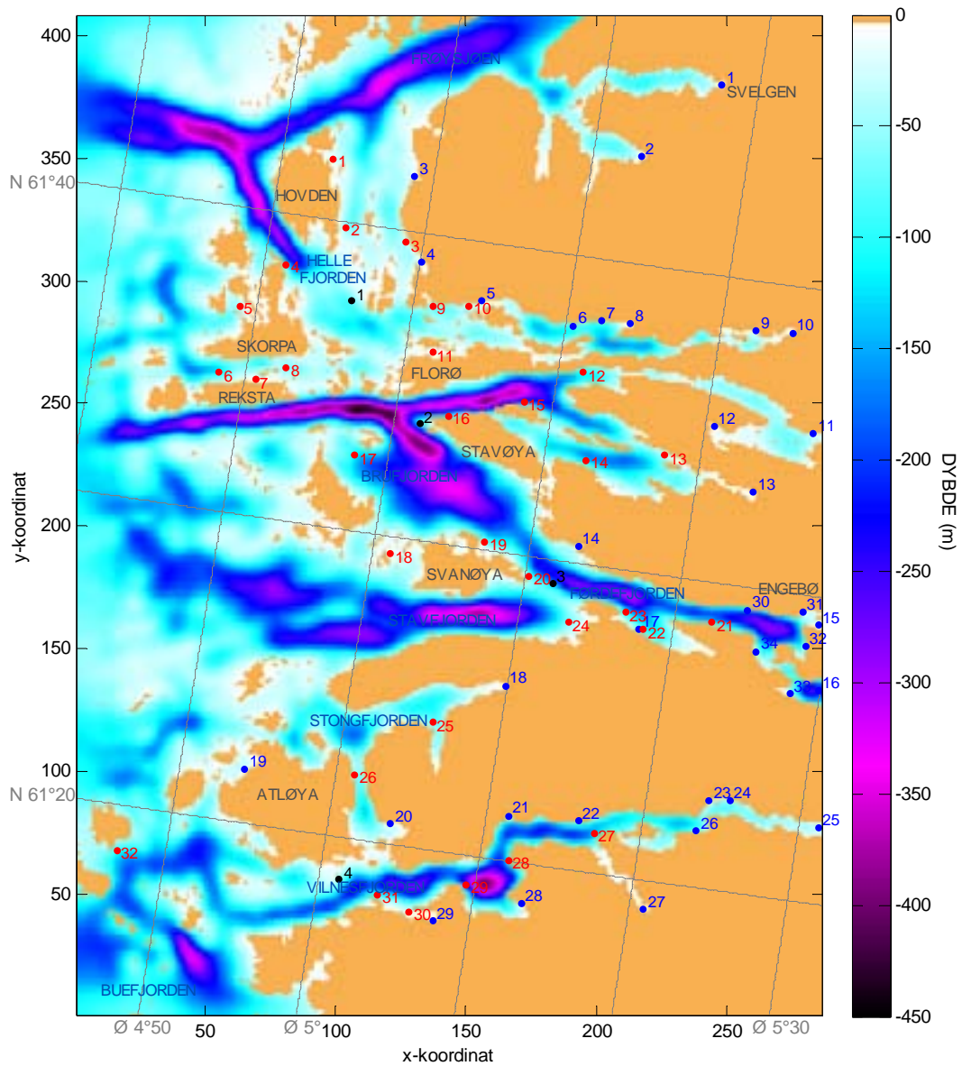
Figur 2. Kart over modellområdet. Oppdrettslokaliteter (røde prikker), elveutløp (blå prikker) og posisjonene til strømmålerne (svarte prikker, nr. 1-4) er tegnet inn. Hver prikk har et identifikasjonsnummer som finnes igjen i posisjonstabellene.
