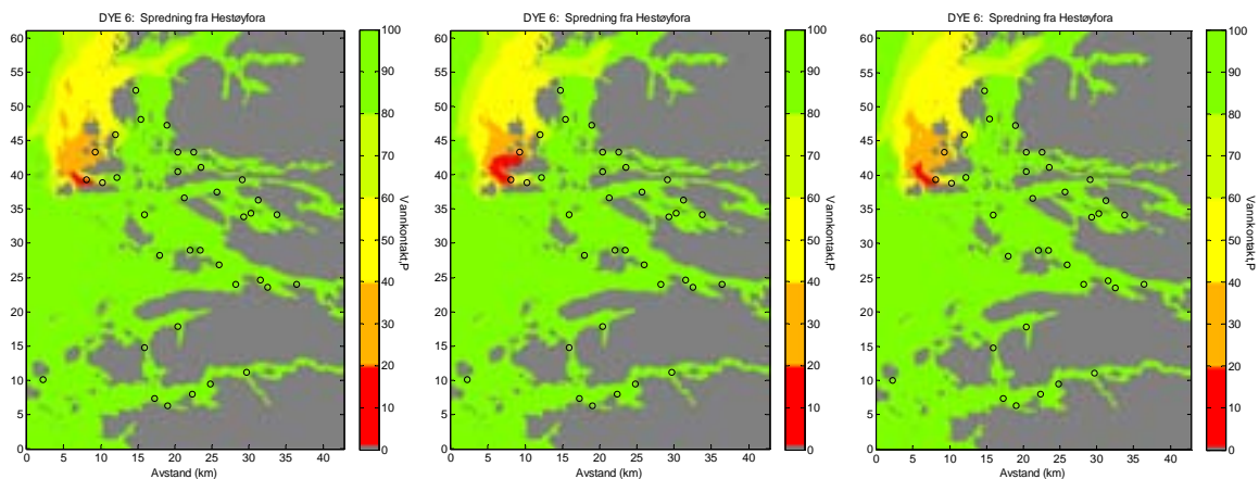
Figur 23. Spredning fra Hestøyfjora. Venstre: Vindstyrken var 5 m/s fra nordvest. Midt: Vindstyrken var 5 m/s fra nordvest og utslippet forsinket med 6 timer. Høyre: Vindstyrken var 5 m/s fra sørvest.
