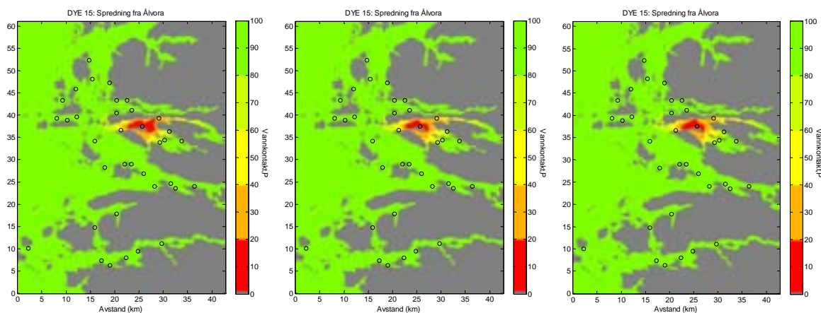
Figur 32. Spredning fra Ålvora. Venstre: Vindstyrken var 5 m/s fra nordvest. Midt: Vindstyrken var 5 m/s fra nordvest og utslippet forsinket med 6 timer. Høyre: Vindstyrken var 5 m/s fra sørvest.
