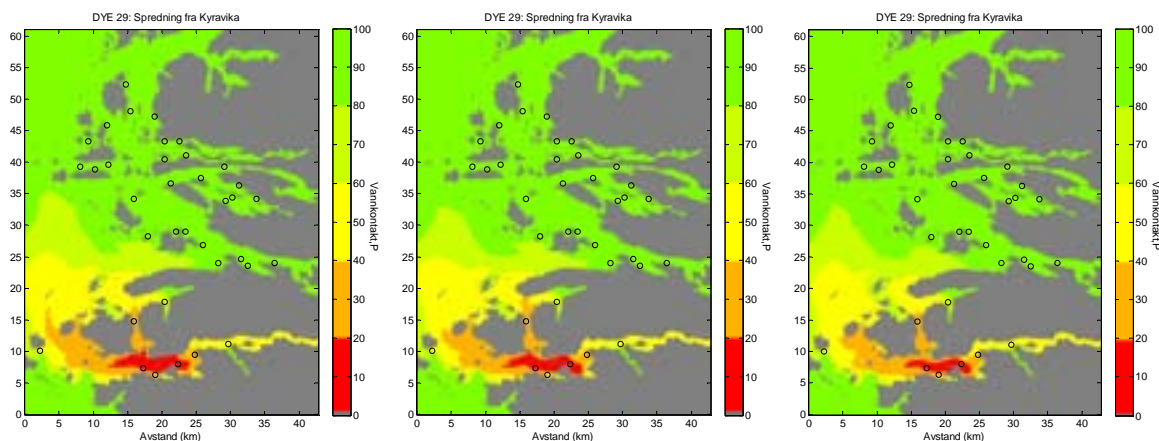
Figur 46. Spredning fra Kyrvika. Venstre: Vindstyrken var 5 m/s fra nordvest. Midt: Vindstyrken var 5 m/s fra nordvest og utslippet forsinket med 6 timer. Høyre: Vindstyrken var 5 m/s fra sørvest.
