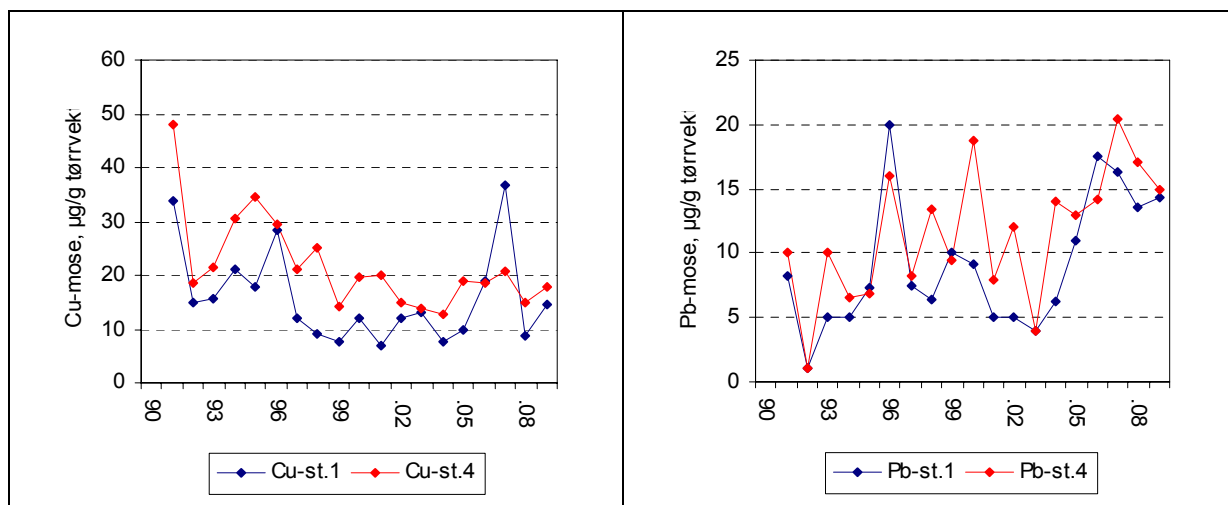
Figur 3. Middelkonsentrasjonene av kobber (Cu) og bly (Pb) i vannmoser ved stasjon 1 (inn i feltet) og 4 (ut av feltet) i Veltmannåa. Fra og med 2006 er konsentrasjonene estimert (se metodekapitlet).
