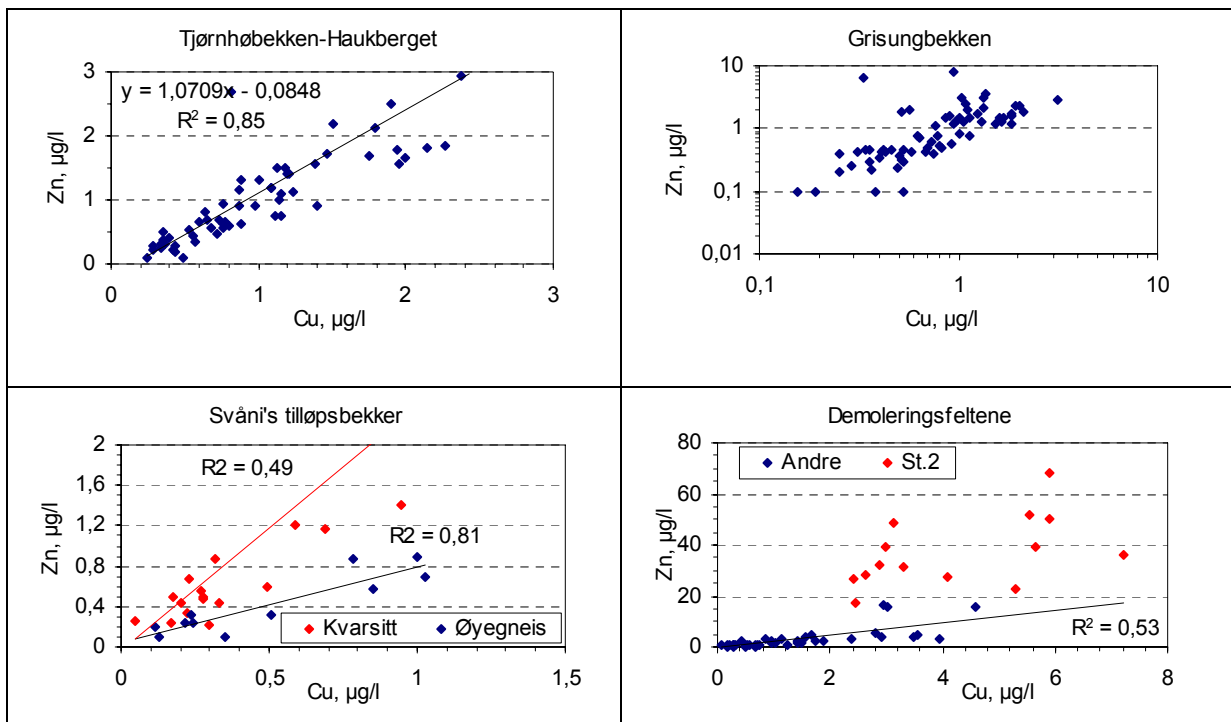
Figur 6. Samvariasjon mellom konsentrasjonene av kobber (Cu) og sink (Zn) i de ulike feltene. Regresjonslinjen for Svani's tilløpsbekker representerer områder bestående av øyegneis, mens linjen for demoleringsfeltene er basert på alle data eksklusive data for st.2 (nedstrøms feltet i Grisungdalen).
