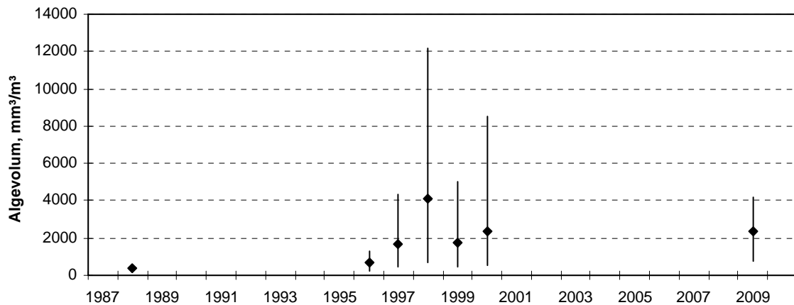
Figur 10. Total algemengde i Gjesåssjøen i 1988, 1996-2000 og i 2009. Figuren viser middelverdier og variasjonsbredder for algeveksts sesongene. Data fra: Faafeng mfl. (1990), Bratli (1998), Berge mfl. (2000 og 2001).
