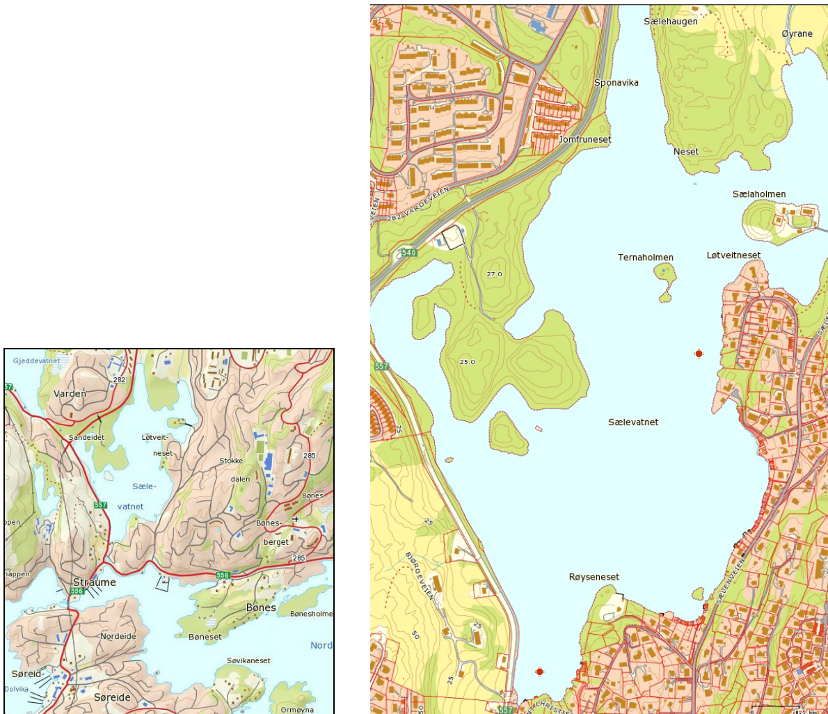
Figur 1. Oversiktskart over Sælenvatnet i Fyllingsdalen, Bergen. I sør ser vi kanalen ut til Nordåsvannet like ved Straume. Sælanelva renner ut i vannet i nord ved Sælehaugen. Måleposisjonene er indikert med røde sirkler.
