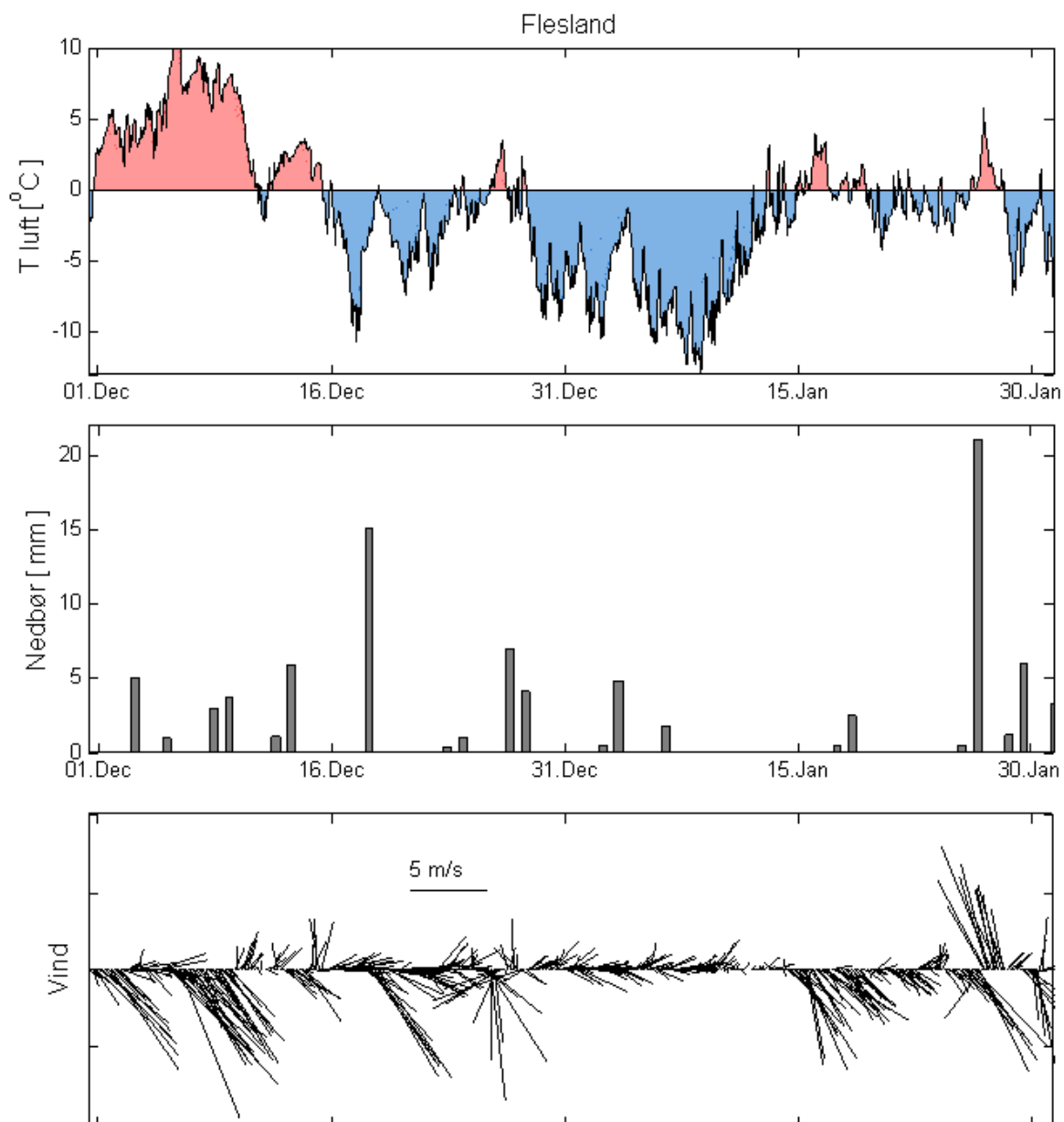
Figur 2. Temperatur (øverst) og vindstyrke med retning (nederst) i perioden desember 2009 til 1. februar 2010. Temperaturen over 0°C er angitt med rød farge, mens blått angir kuldegrader. Vinden er indikert med piler (streker) som gir både retning og styrke. Vinden er midlet over 6 timer. Data hentet fra eklimate.no.
