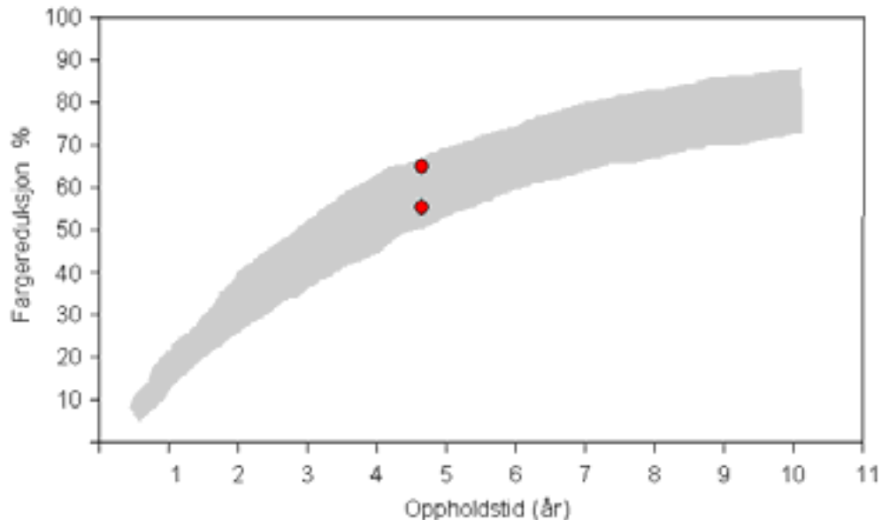
Figur 21. Antatt forløp som viser fargereduksjoner i innsjøer som funksjon av oppholdstiden. De 2 punktene viser farge-reduksjon i Glitre ved 2 datasett: 1998-2001 og 2002-2003, hhv 65 % og 55 % reduksjon (Berge og medarb 2004).
