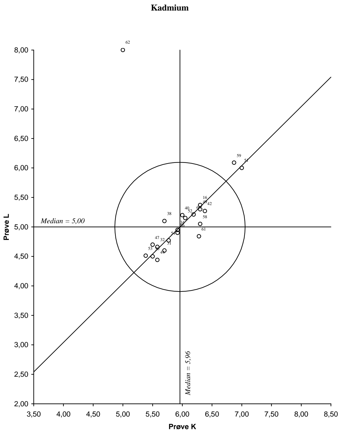
Figur 42. Youdendiagram for kadmium, prøvepar KL Akseptansegrensen, angitt med en sirkel, er 20 %
