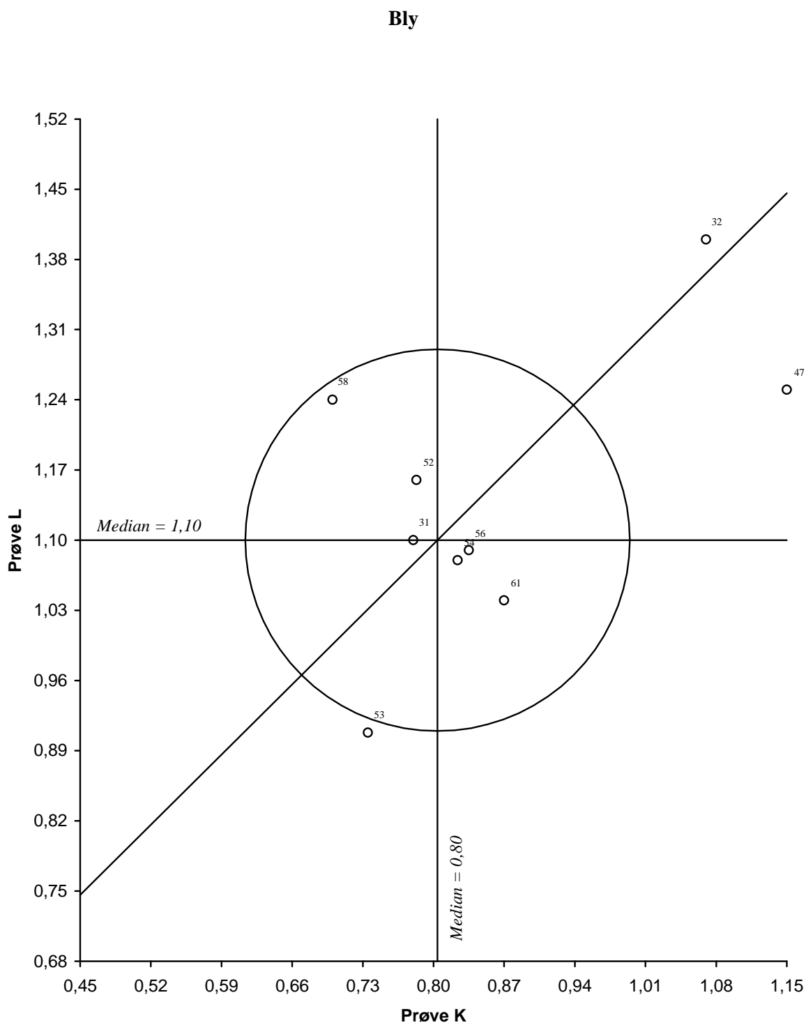
Figur 38. Youdendiagram for bly, prøvepar KL Akseptansegrensen, angitt med en sirkel, er 20 %
