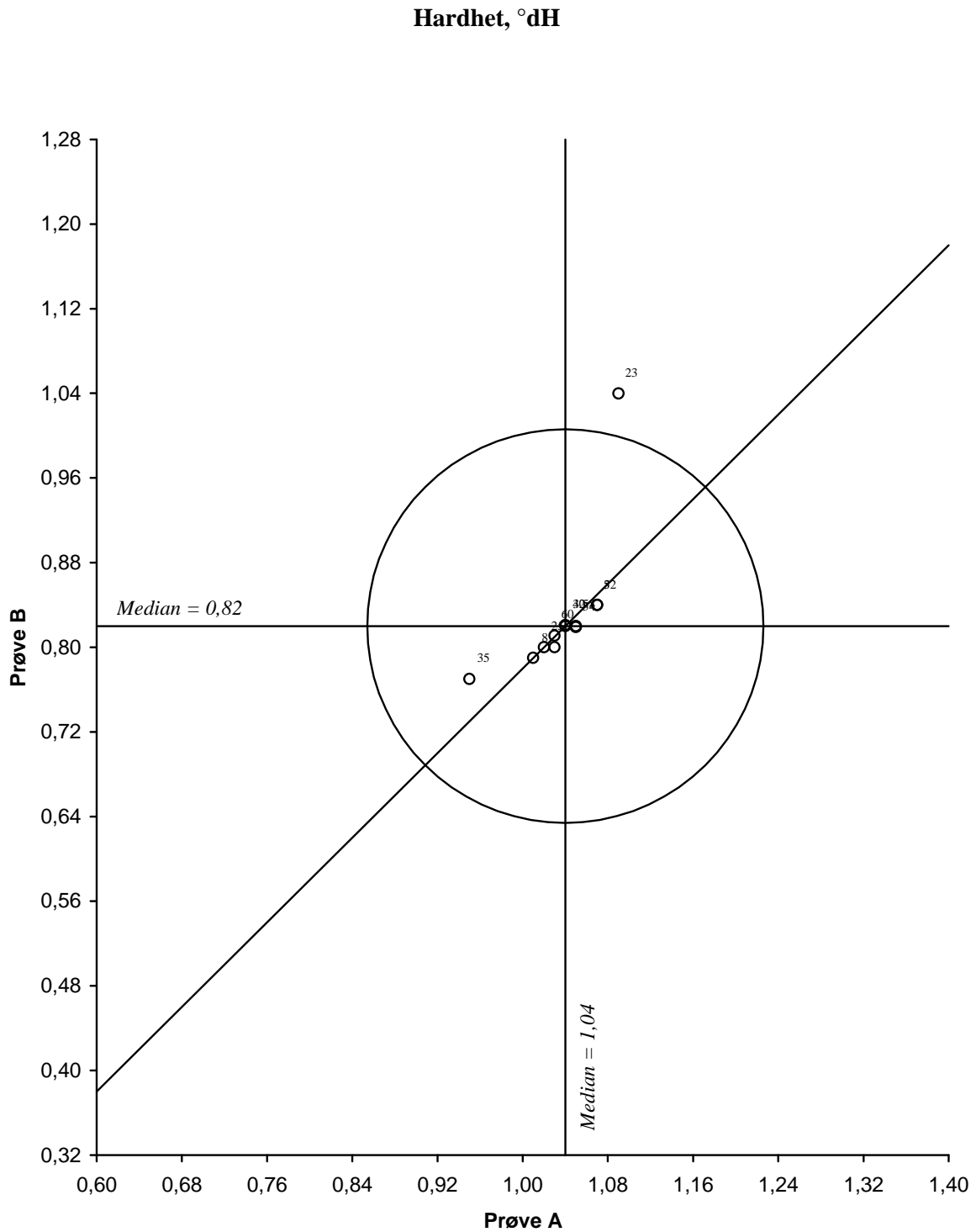
Figur 13. Youdendiagram for hardhet, prøvepar AB Akseptansegrensen, angitt med en sirkel, er 20 %
