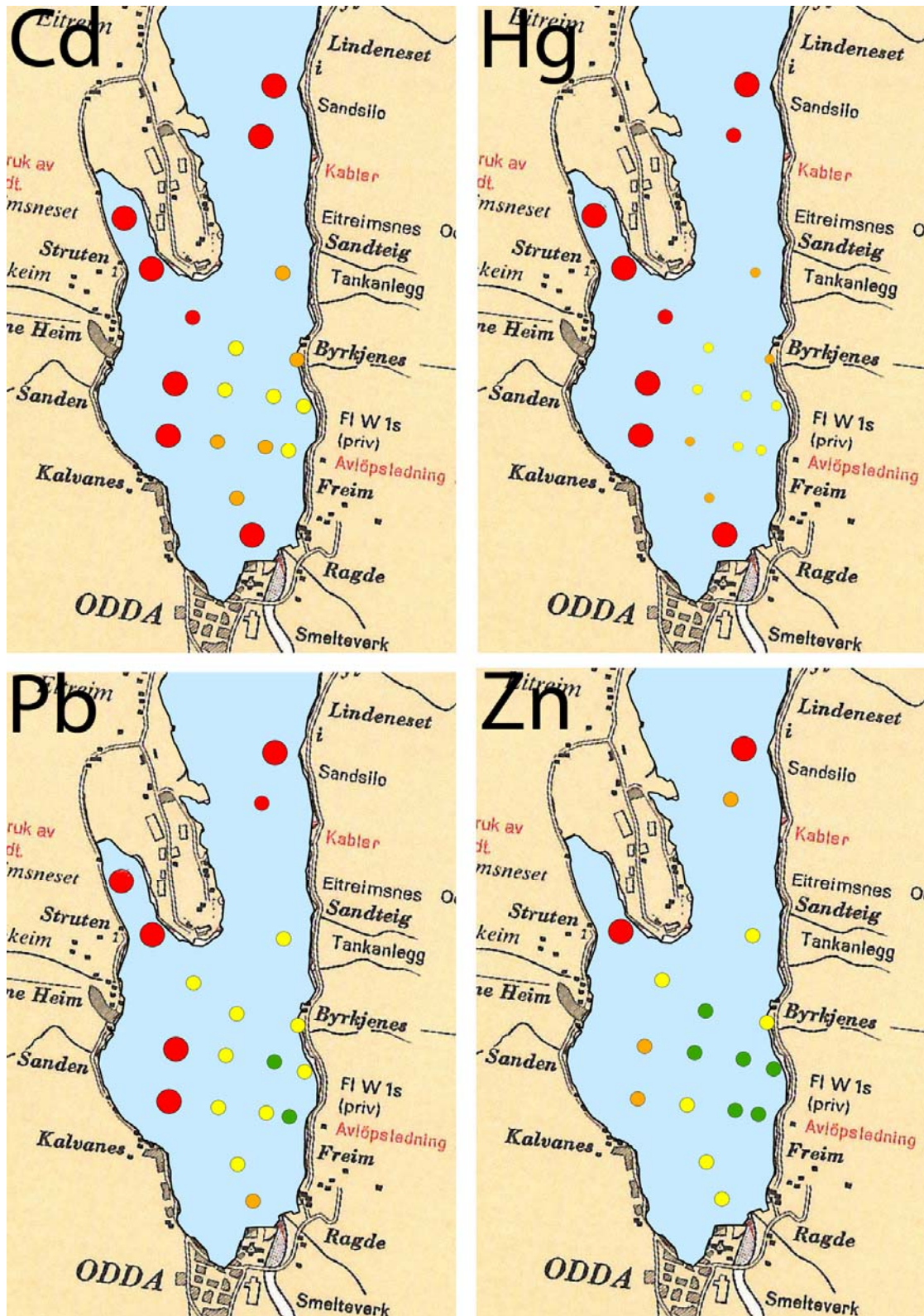
Fig.12. Nivåer av metaller i overflatesedimentene i indre Sør fjorden. Fargene på sirklene indikerer SFTs tilstandklasser hvor rød er kl.V. Store røde sirklene indikerer sedimenter med ekstremt høye nivåer (flere ganger øvre grense for kl V).
