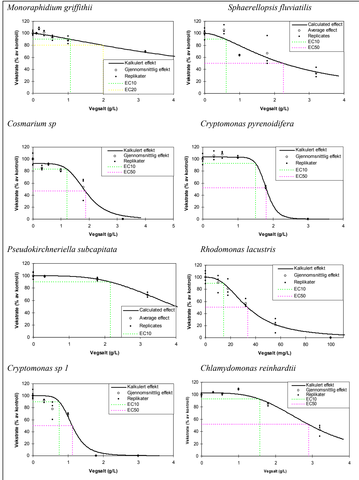
Figur 133. Vekstrate med EC10 og EC50 verdier for ulike testalger i en konsentrasjonsrekke av vegsalt.
