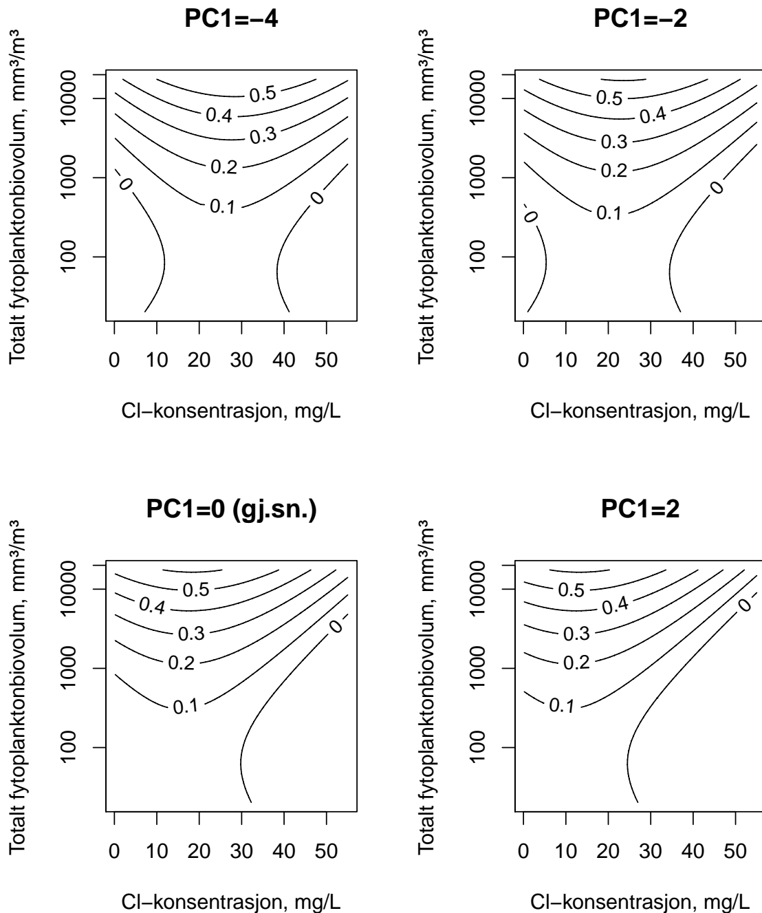
Figur 9. Predikert andel av blågrønnalger (isokliner) som funksjon av kloridkonsentrasjon, totalt biovolum av planktonalger samt prinsipalkomponent 1 (PC1). Lave PC1-verdier angir økende grad av kalkrikhet. PC1=0 angir en gjennomsnittlig vannkjemi. Prediksjonene er generert fra GAM i Tabell 7, Vedlegg A. Modellen forklarer 28 % av variasjonen.
