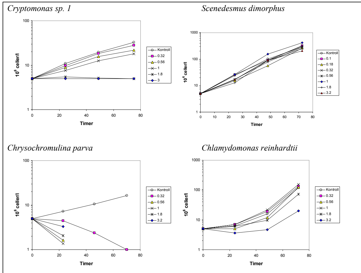
Figur 144.. Gjennomsnittlig celletetthet gjennom testene. Legg merke til at y-aksen er logaritmisk.
