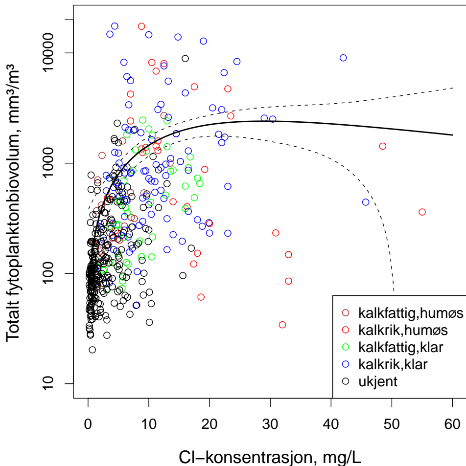
Figur 1. Biplott av relasjonen mellom klorid og total planktonalgebiovolum. Typologi er indikert med egne farger på punktene. Merk at y-aksen er \log_{10} -transformert. Prediksjonslinja og tilhørende 95 % konfidensintervall er fra GAM-modell med 2.2 estimerte frihetsgrader der 11 % av variasjonen forklares av modellen.
