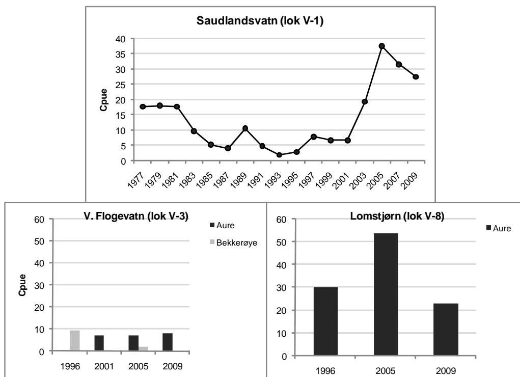
Figur 51. Fangst av aure pr. 100 m 2 garnareal (Cpue) i bunnære områder (0-12 m dyp) av Saudlandsvatn og Lomstjørn og av aure og bekkerøye i V. Flogevatn i ulike perioder.
