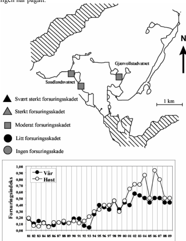
Figur 65. Oversikt over innsamlingslokaliteter og sammensetning av bunndyr i Farsund-området i 2009. Figuren viser også gjennomsnittlige forursingsverdier vår (V) og høst (H) i perioden 1981-2009.
