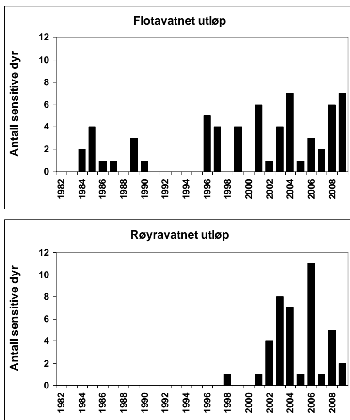
Figur 60. Forekomst av forsuringssensitive bunndyr i utløpselvene fra Flotavatnet og Røyrvatnet (Vikedal) i perioden 1982-2009.
