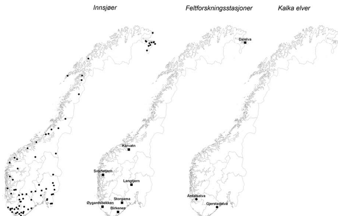
Figur 8. Lokalisering av alle de undersøkte lokalitetene i 2009 (innsjøer, elver og feltforskningsstasjoner). Linjene viser grensen til de 10 regionene (se Vedlegg A for inndeling av regioner).
