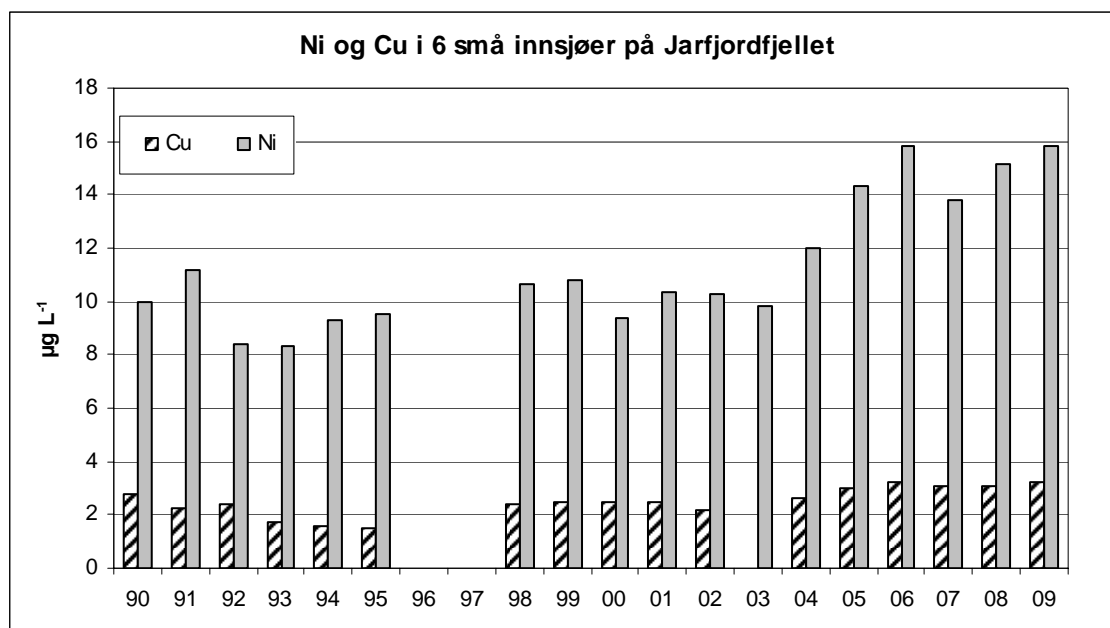
Figur 27. Årlige middelerdier for nikkell og kobber i seks små innsjøer på Jarfjordfjellet fra 1990 til 2009.
