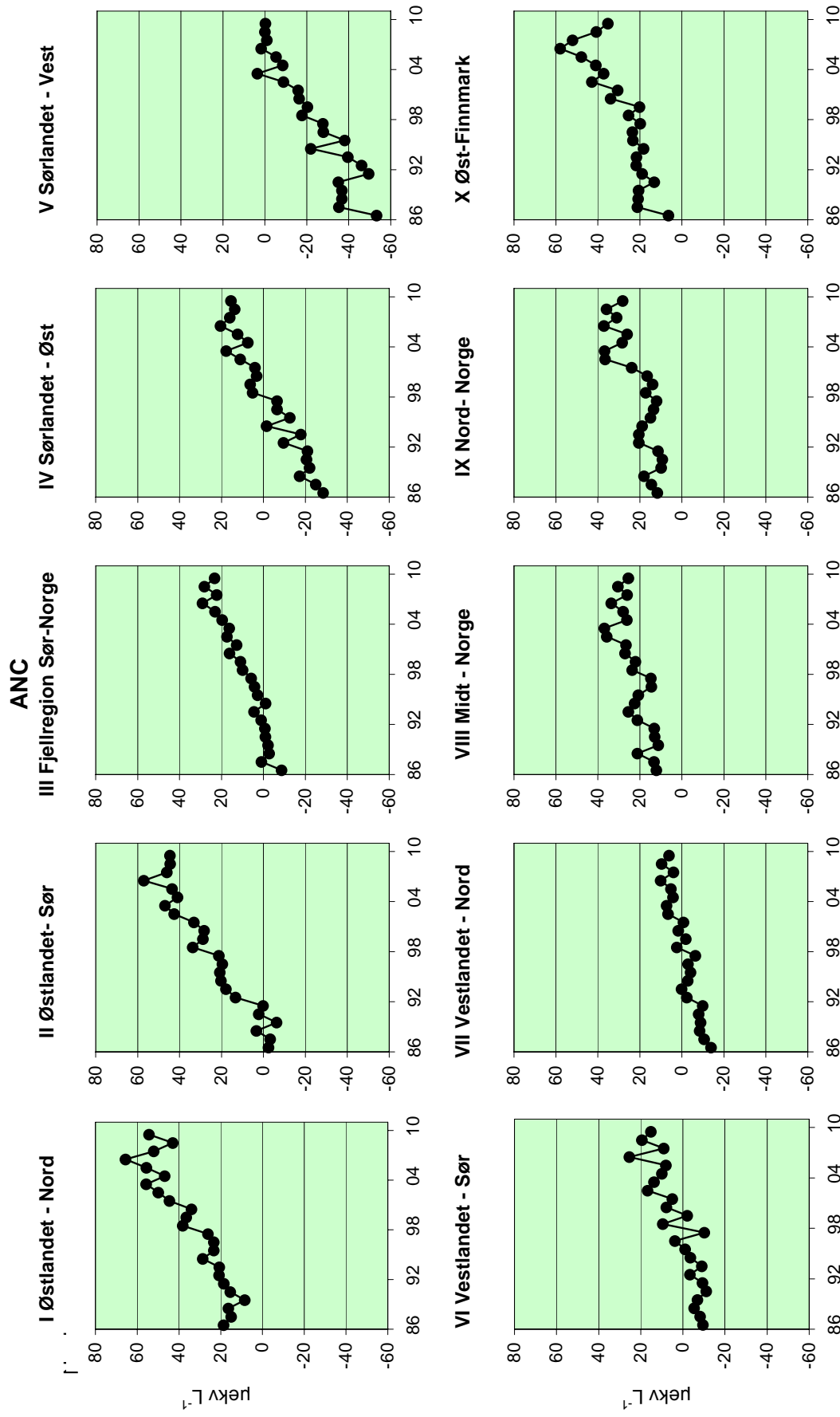
Figur 21. Trender for perioden 1986-2009 for ANC (syrenøytraliserende kapasitet) for innsjøer i de 10 regionene.
