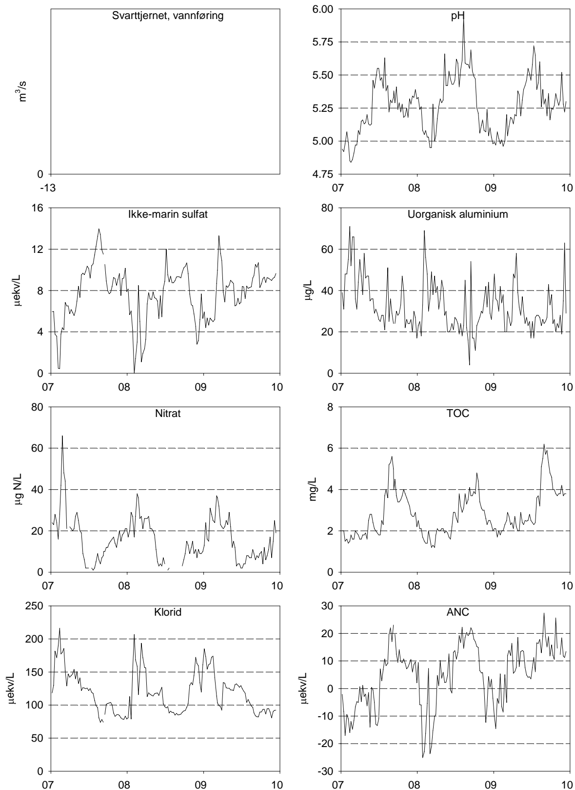
Figur 14. Sesongvariasjon i avrenning og konsentrasjon for ulike vannkjemiske parametere i Svarttjernet i perioden 2007-2009. OBS! Ingen vannføringsstasjon
