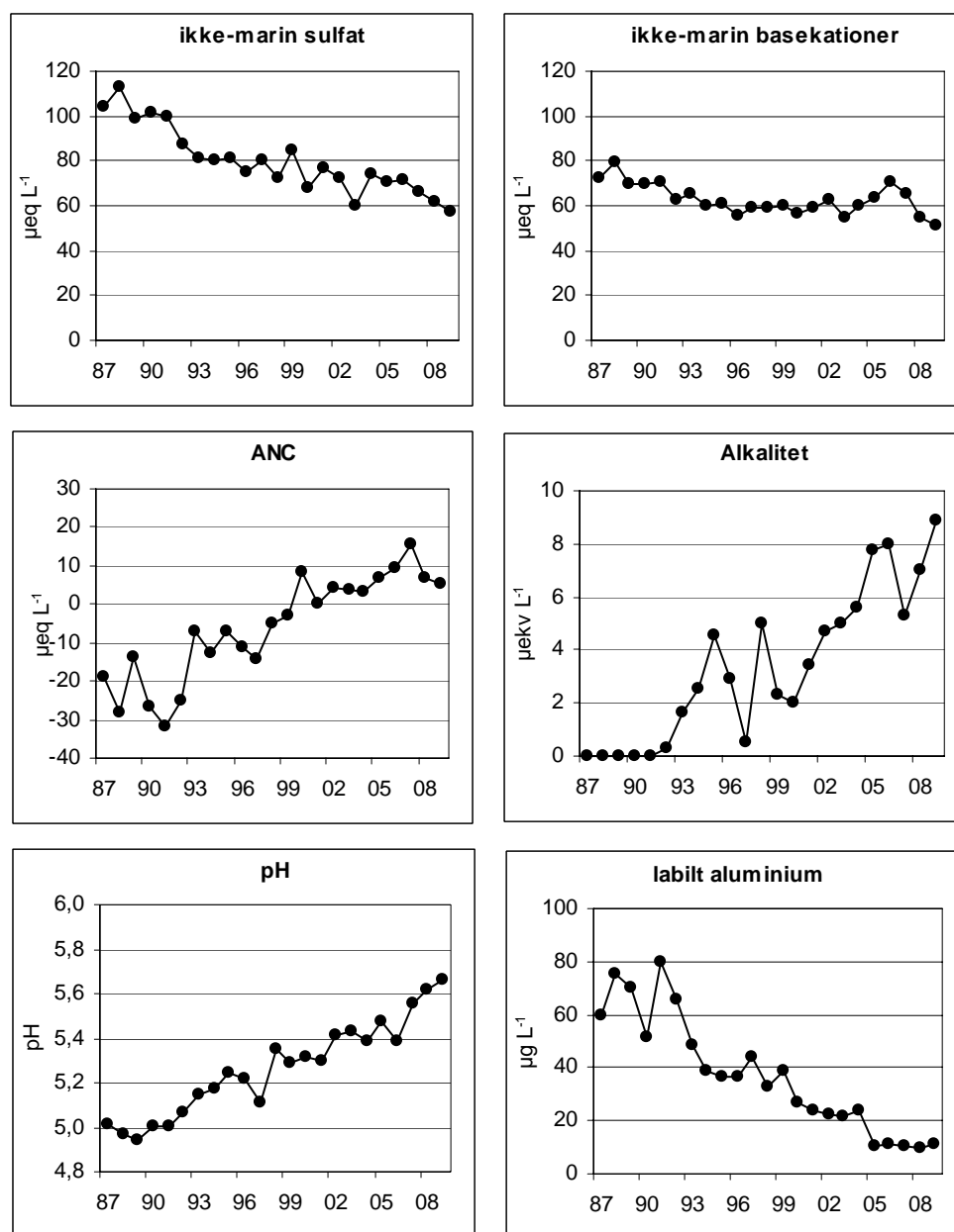
Figur 26. Forsuringsparametre for seks små vann på Jarfjordfjellet i 1987-2009. Middelerverdier for ikke-marine basekationer ( BC^* ), ikke-marin sulfat ( SO_4^* ), ANC, alkalitet, pH og labilt aluminium.
