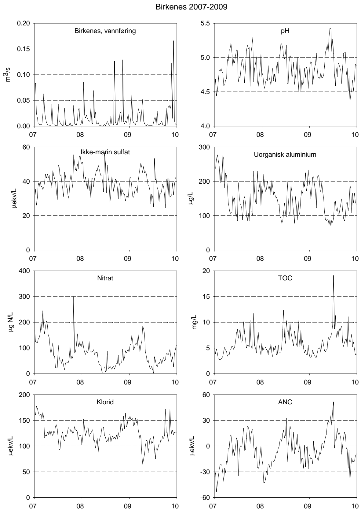
Figur 9. Sesongvariasjon i avrenning og konsentrasjon for ulike vannkjemiske parametere i Birkenes i perioden 2007-2009.
