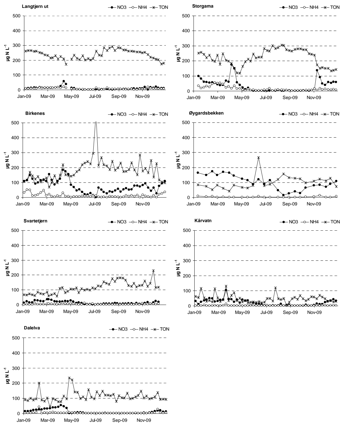
Figur 42. Sesongmessig fordeling av nitrat ( \text{NO}_3 ), ammonium ( \text{NH}_4 ) og totalt organisk nitrogen (TON) i feltforskningsområdene i 2009. TON = total nitrogen – \text{NO}_3 – \text{NH}_4 . Enhet: \mu\text{g N L}^{-1} .
