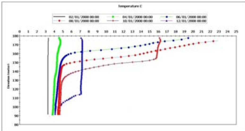
Figur 11. Eksempler på vertikal fordeling av temperatur nær vanninntaket i løpet av året i følge simulerte verdier 2008 over det dypeste partiet i vestre del av Birkelandsvann (Storavatn).
