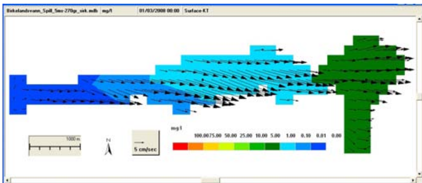
Figur 36. Vind 5 m/s fra Vest. Utlipp 10 \text{ m}^3/10 \text{ tonn} i øst. Konsentrasjoner etter to dager på overflaten.
