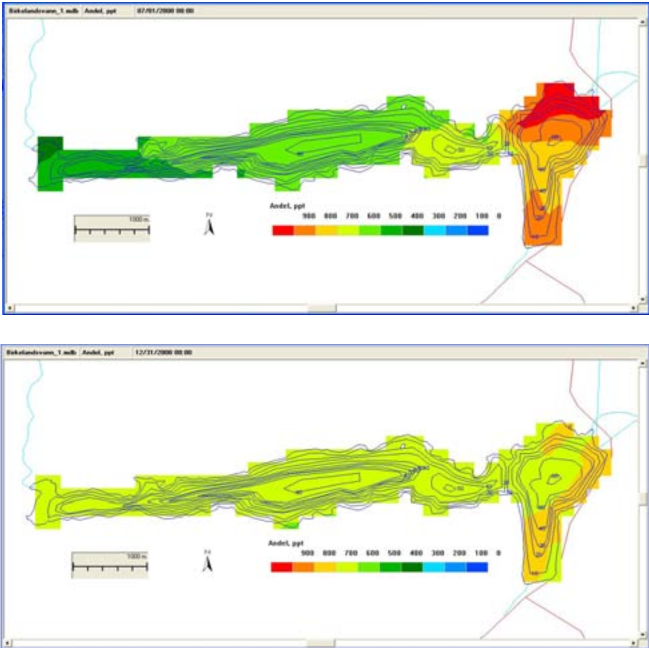
Figur 15. Overflate. Innblanding av vann tilført østre basseng etter 6 måneder og 12 måneder i 2008.
