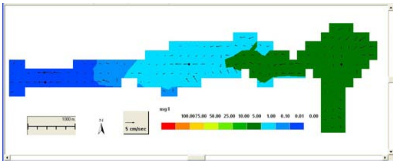
Figur 37. Vind 5 m/s fra Vest. Utlipp 10 \text{ m}^3/10 \text{ tonn} i øst. Konsentrasjoner etter to dager langs bunnen.
