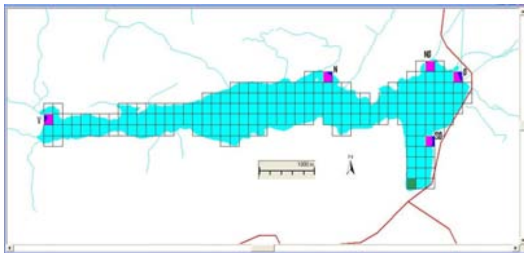
Figur 1. I modellen ble innsjøen delt inn i beregningsceller, 160 m · 180 m i horisontalplanet og 1 meter i dybderetningen. Det ble antatt fire tilførselspunkter (røde) og ett utløp (grønt) i overflaten. I tillegg ble det plassert et dypvanninntak nær dypeste punkt i vestre eller østre del.
