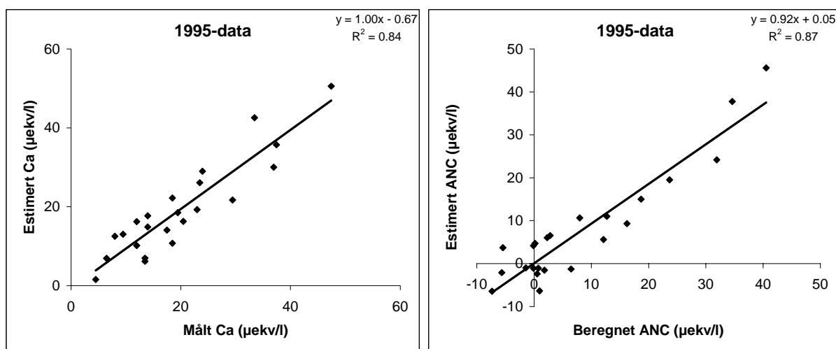
Figur 3. Validering av modell ved korrelasjon av målt og estimert Ca-konsentrasjon (venstre panel) og beregnet og estimert ANC (høyre panel). Data fra alle 1995-innsjøer i den nordvestre delen av Sogn og Fjordane (med unntak av en utligger) med Cl-konsentrasjon <12 mg/l og Ca/Mg-forhold <8 (46), hvorav data fra 23 innsjøer er brukt til å lage modellen og data fra de 23 resterende innsjøene til validering av modellen.
