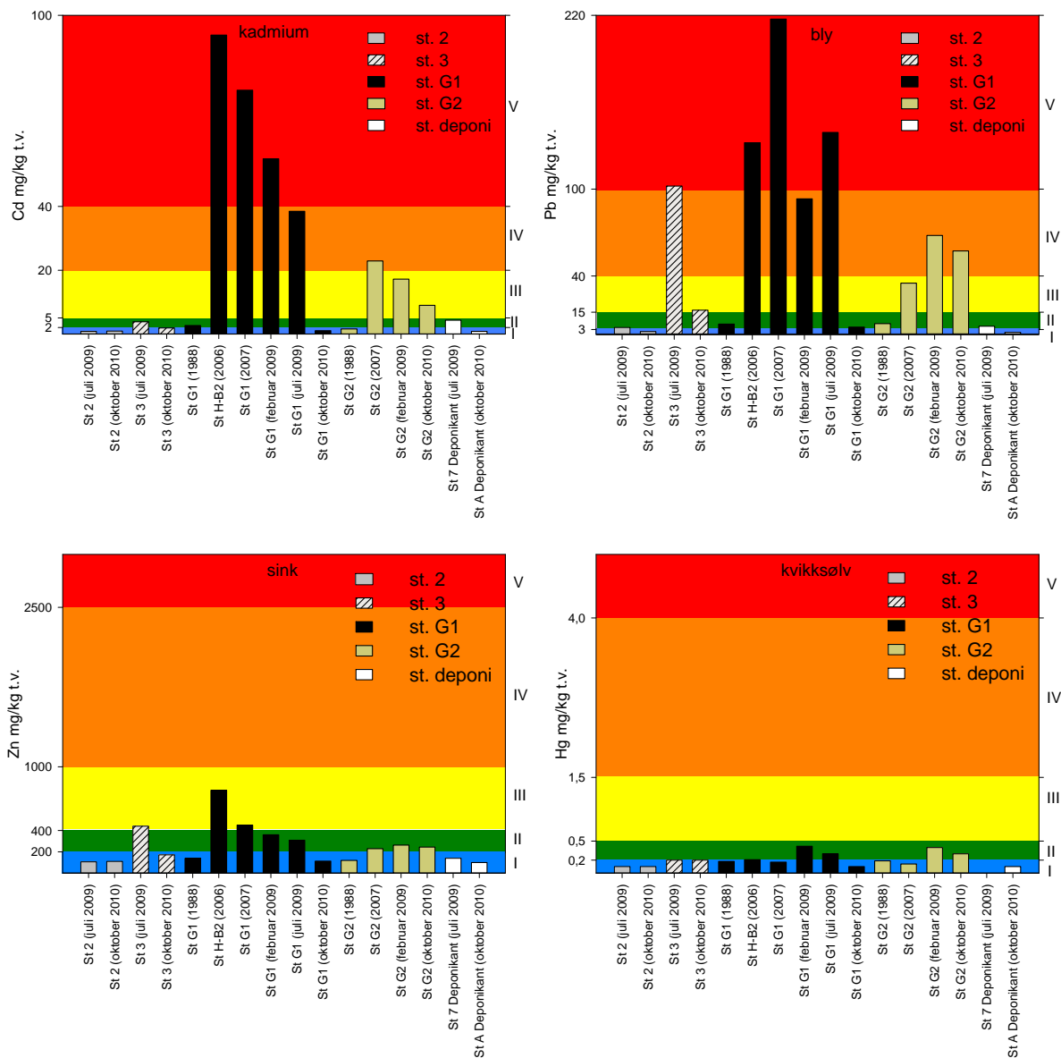
Figur 4. Metallinnhold i blåskjell fra 5 stasjoner i Høyangsfjorden, (stasjon HB-2 2006 ligger nær stasjon G1 og er sammenlignet med denne). Fargekode og romertall tilsvare Klif's tilstandsklasser.
